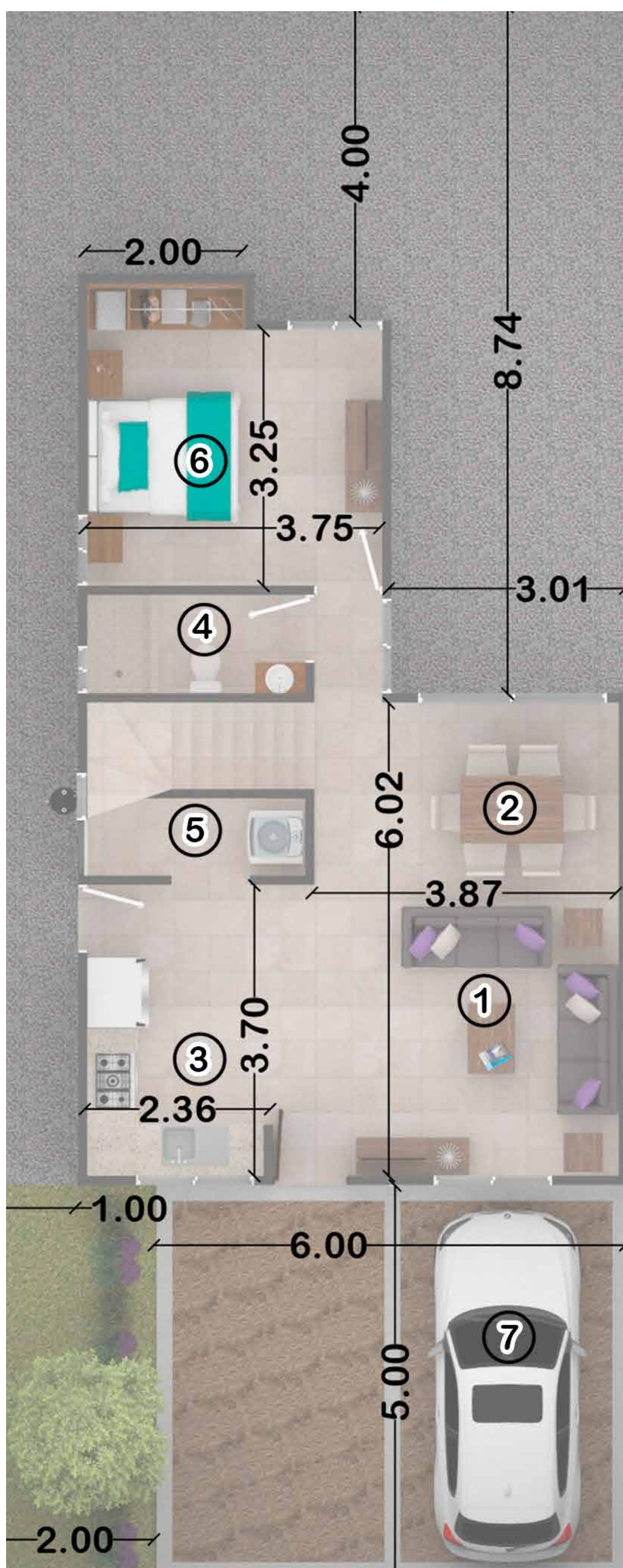
Planta Baja
