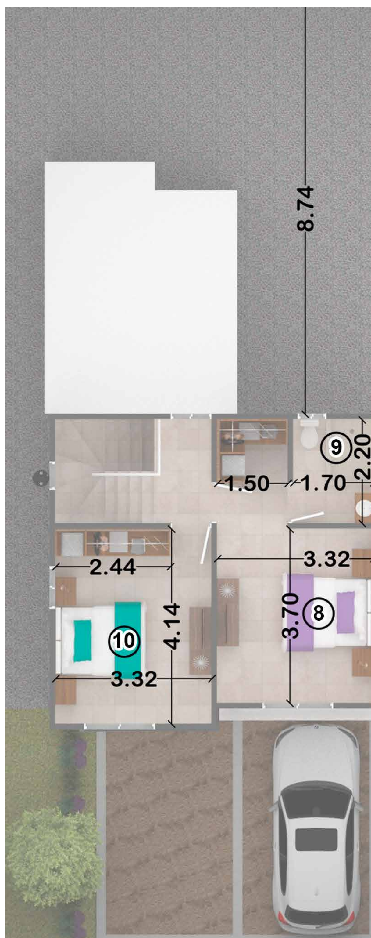
Planta Alta
