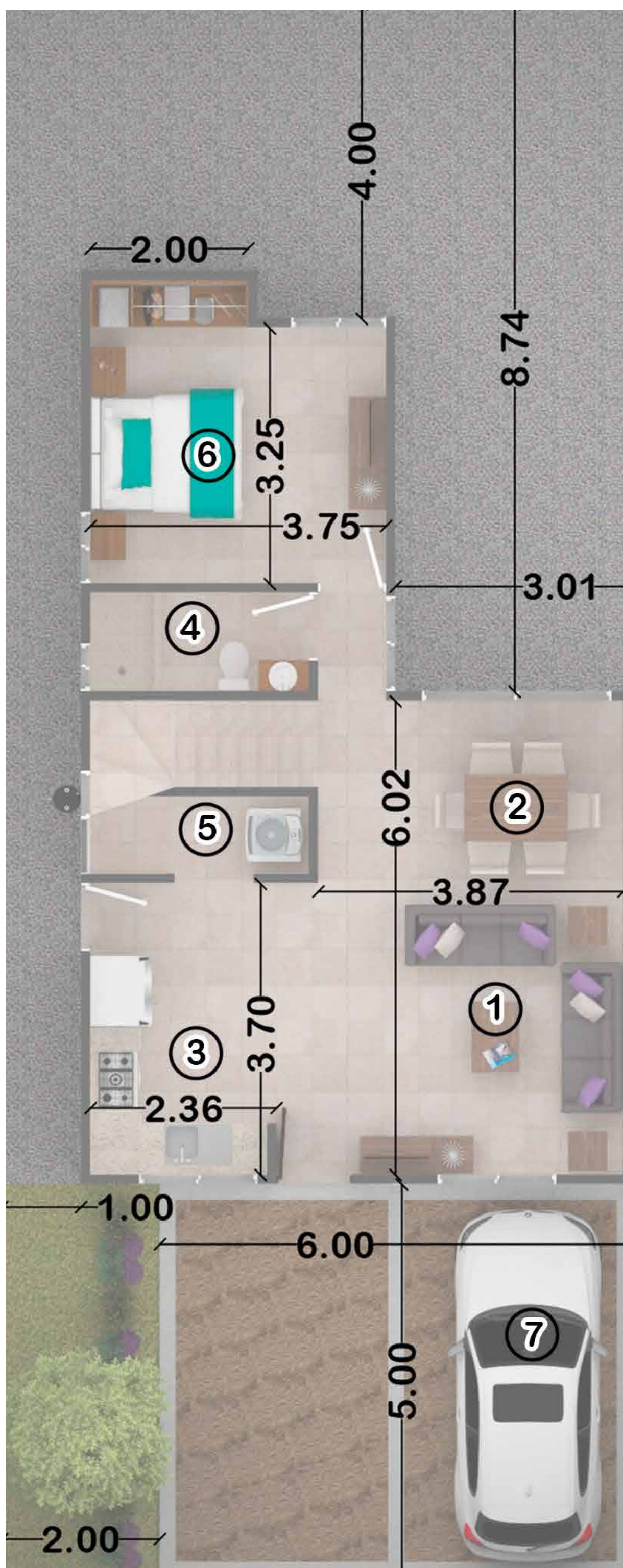
Planta Baja
