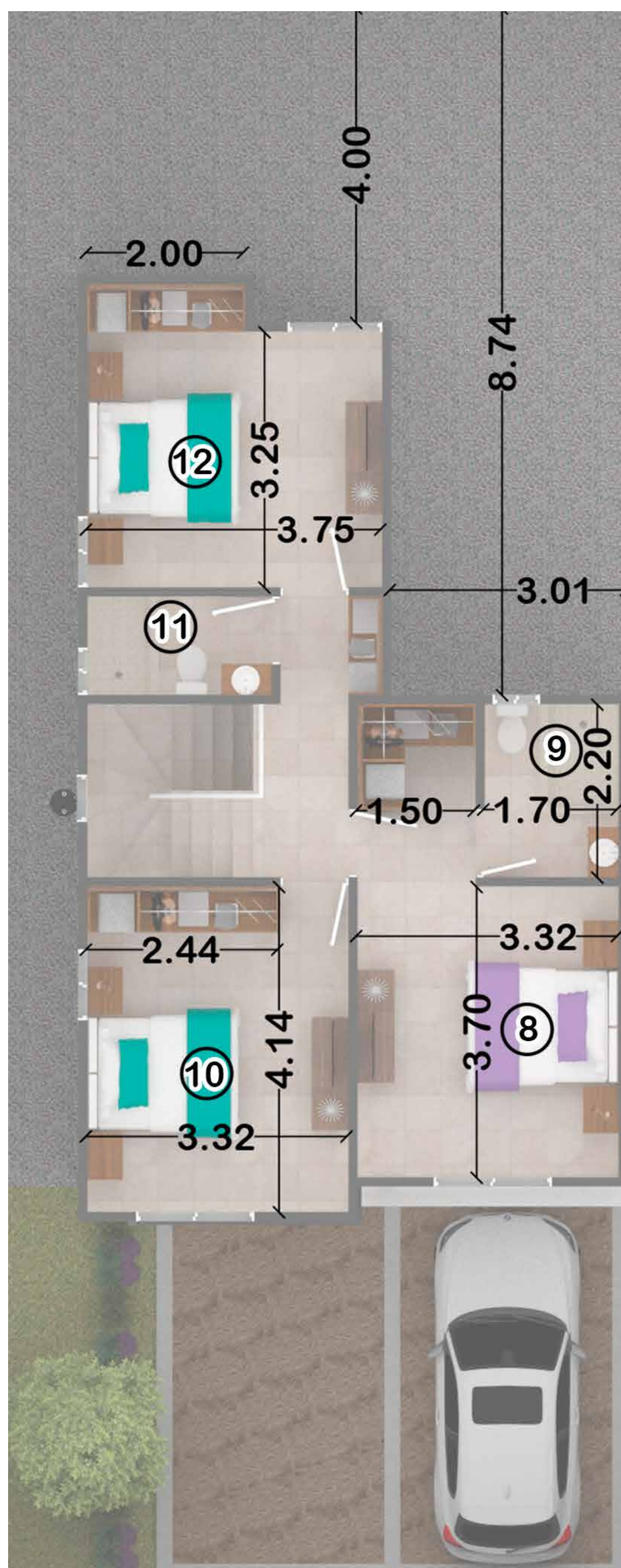
Planta Alta
