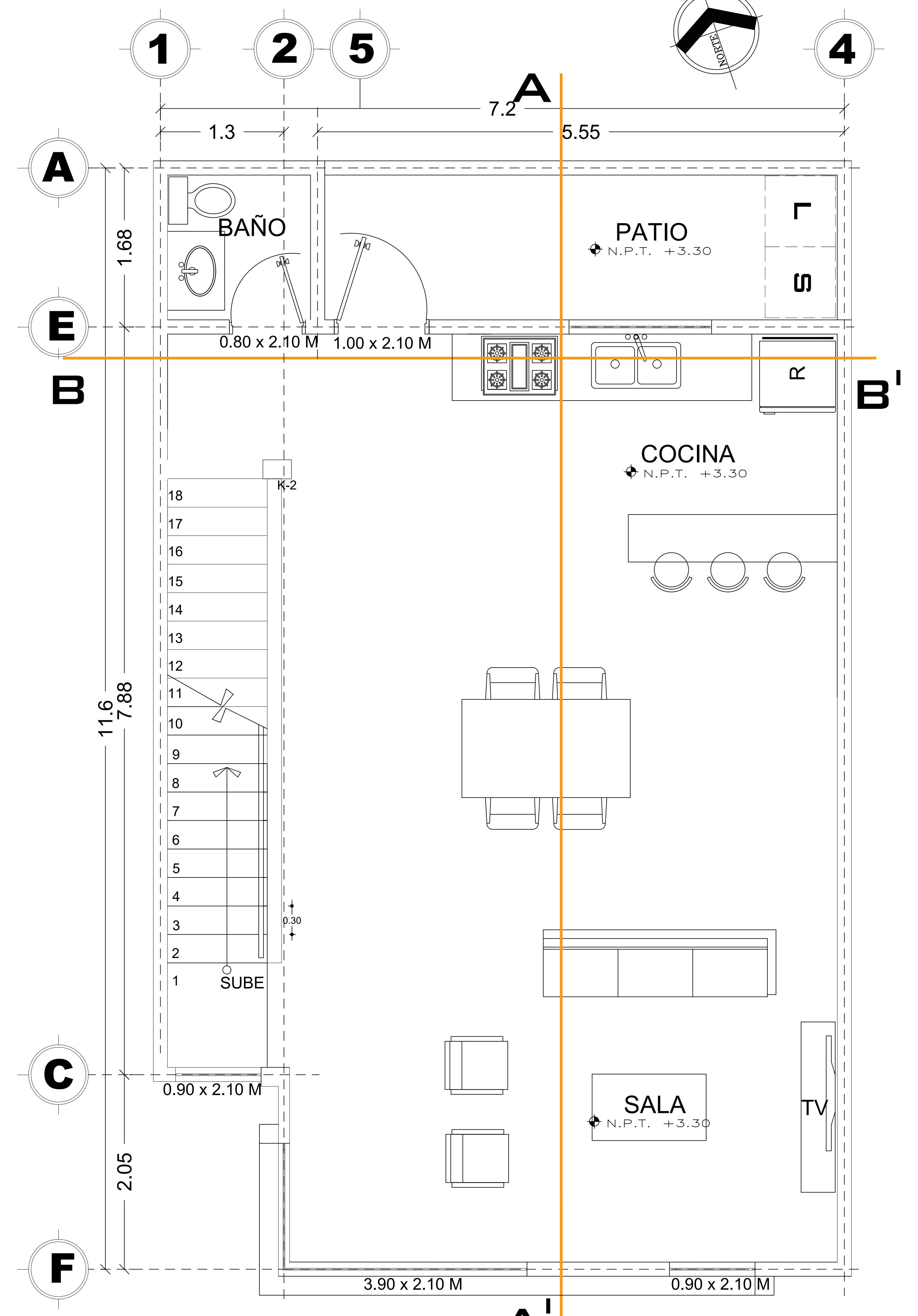
2 PLANTA 1ER NIVEL ESC 1:50
