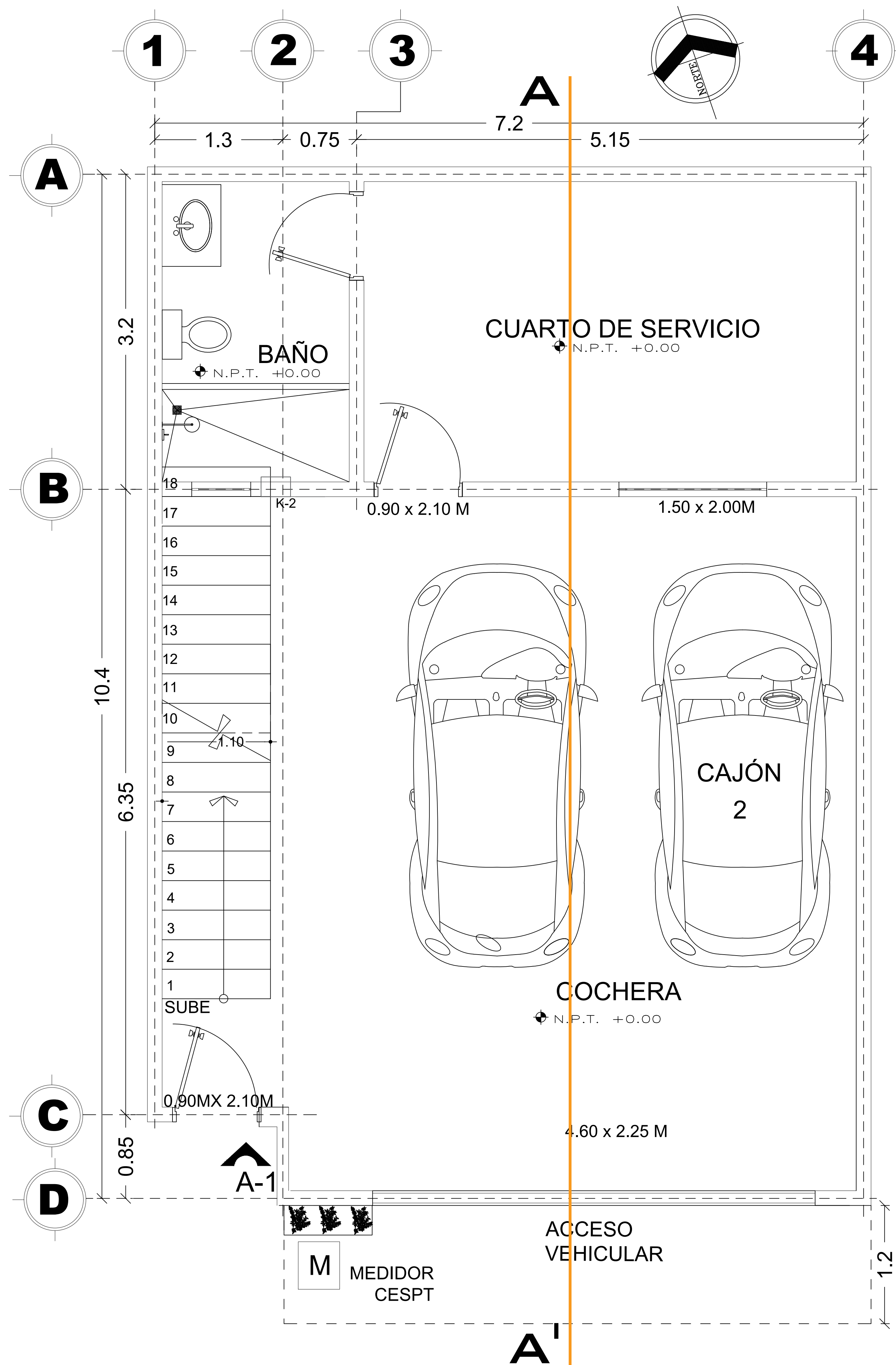
1 PLANTA BAJA ESC 1:50
