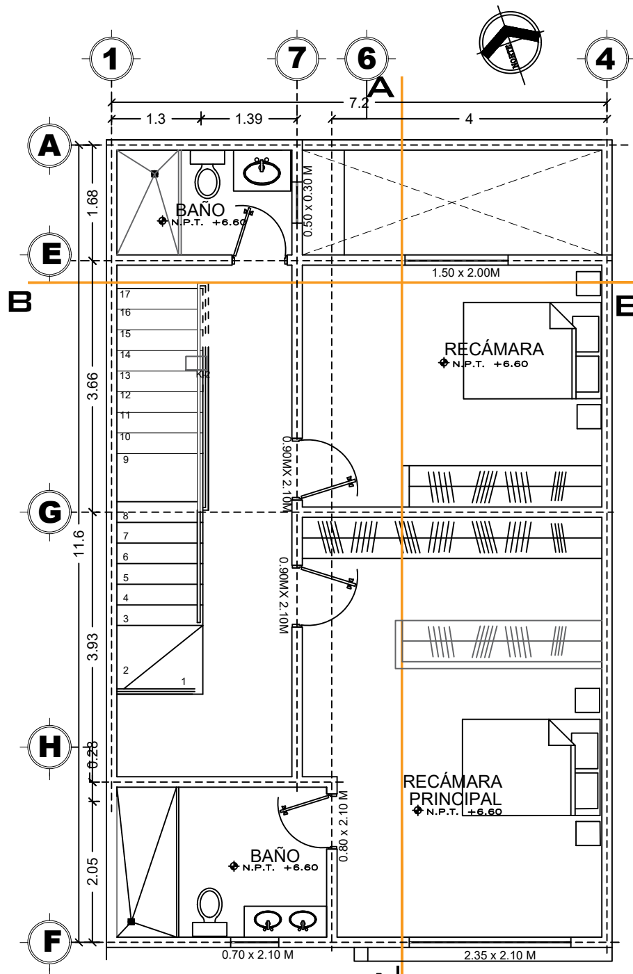
3 PLANTA 2DO NIVEL ESC 1:50
