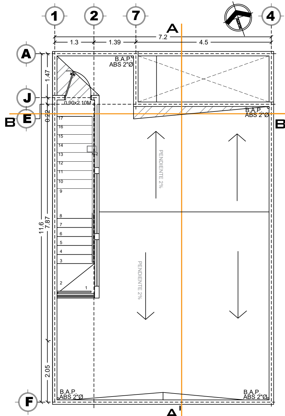
4 PLANTA DE CONJUNTO ESC 1:50
