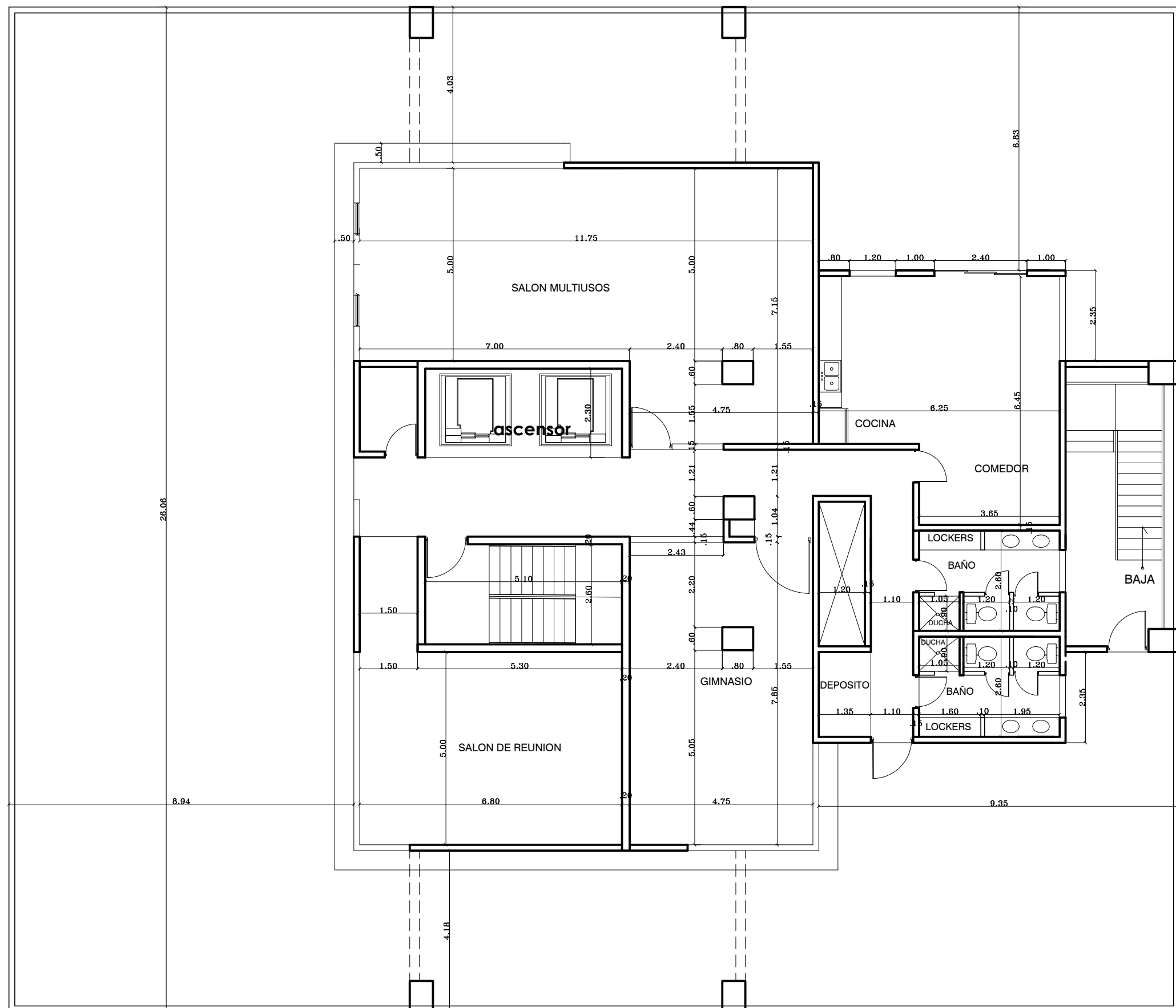
PLANTA ARQUITECTONICA DIMENSIONADA DECIMO
