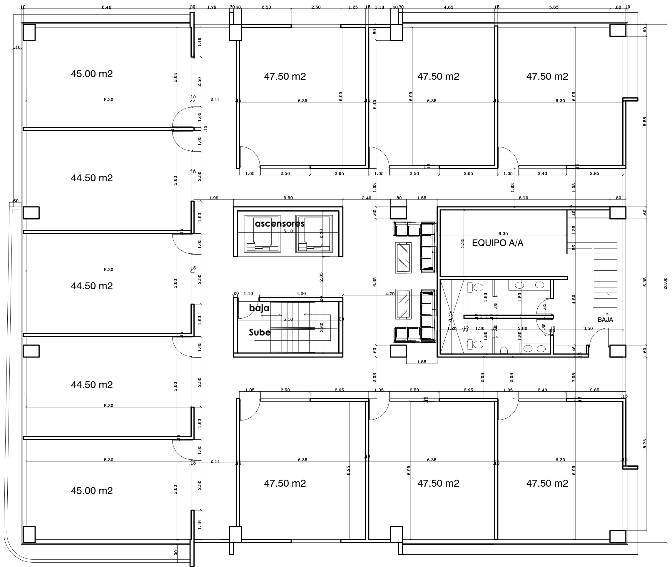
PLANTA ARQUITECTONICA DIMENSIONADA 2DA HASTA 9NO PISO
