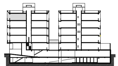
CORTE ESQUEMÁTICO
