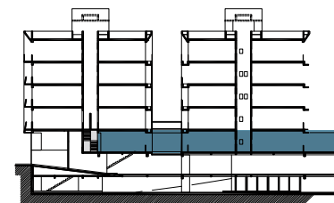
CORTE ESQUEMÁTICO
