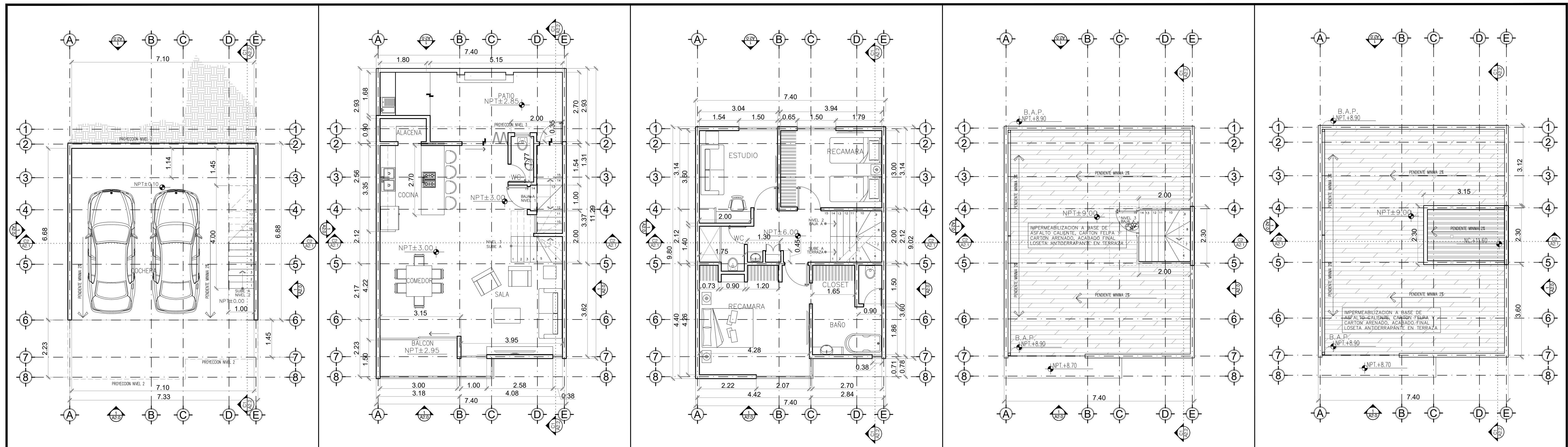
A NIVEL 1 PLANTA TIPO COCHERA ESCALA: 1:75 B NIVEL 2 PLANTA TIPO SALA COMEDOR COCINA ESCALA: 1:75 C NIVEL 3 PLANTA TIPO RECAMARAS ESCALA: 1:75 D NIVEL 4 PLANTA TIPO TERRAZA ESCALA: 1:75 E NIVEL 4 PLANTA TIPO CUBIERTA ESCALA: 1:75
