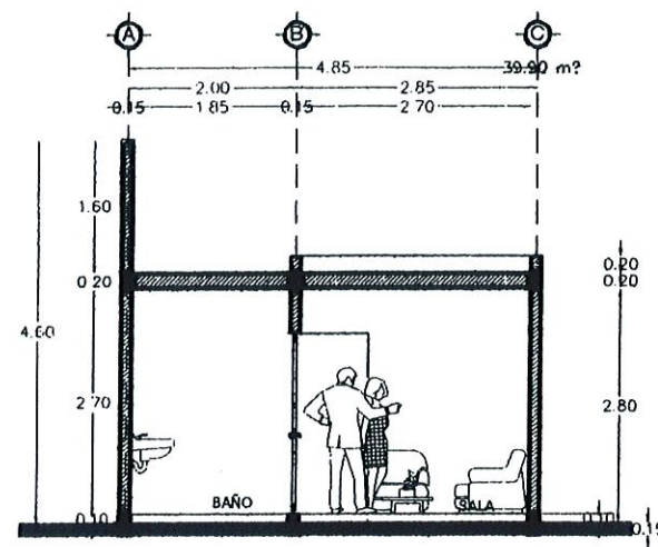
CORTE A-A' VIVIENDA TIPO
