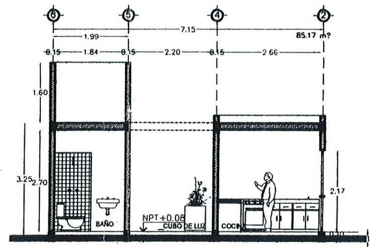
CORTE B-B' VIVIENDA TIPO
