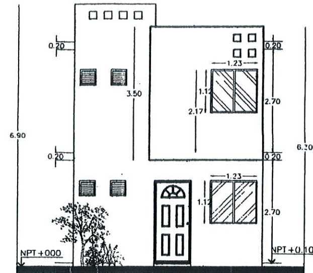
FACHADA 1era.ETAPA CRECIMIENTO
