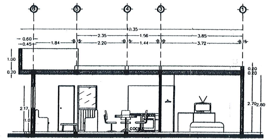
CORTE C-C' VIVIENDA TIPO
