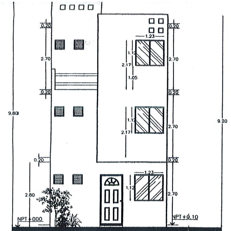
FACHADA 2a.ETAPA CRECIMIENTO
