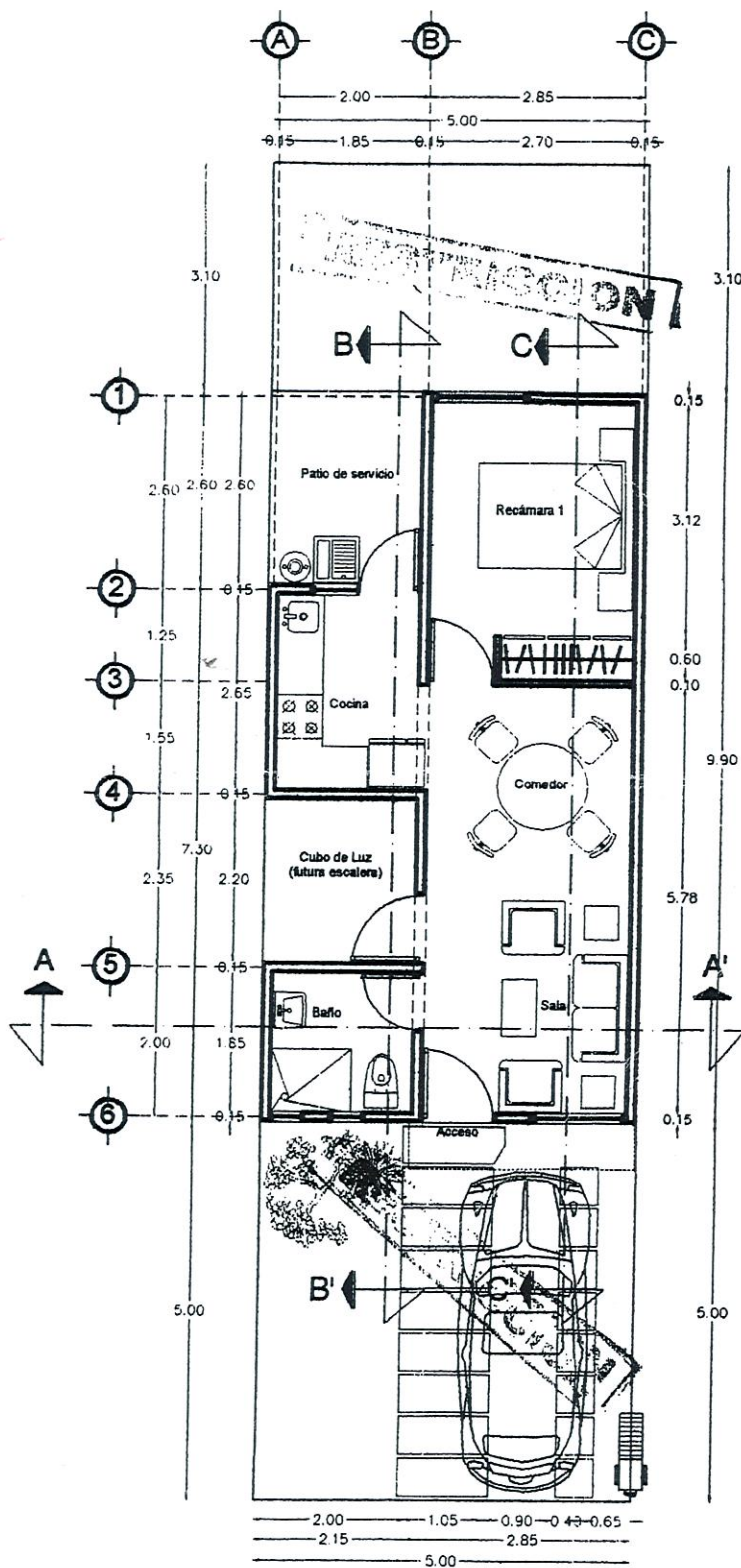
PLANTA ARQUITECTONICA VIVIENDA TIPO 39.90 M2
