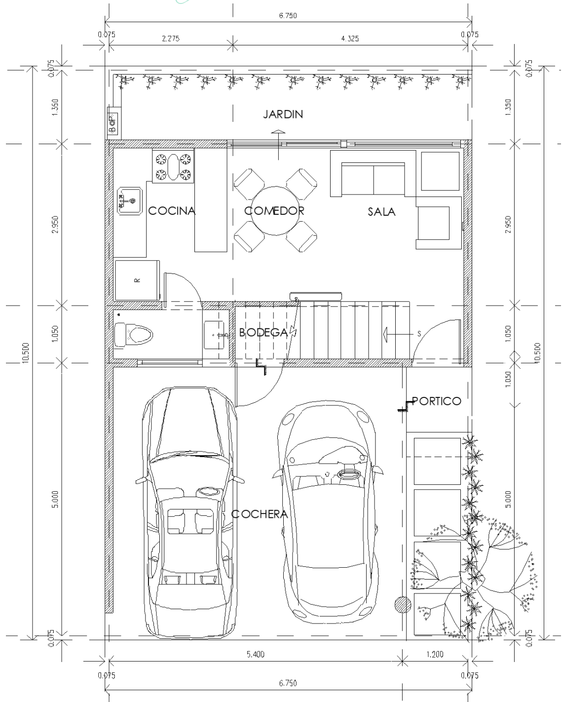
PLANTA BAJA
