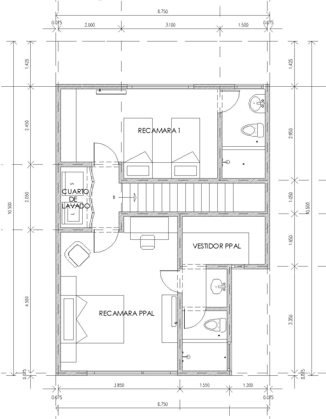
PLANTA ALTA
