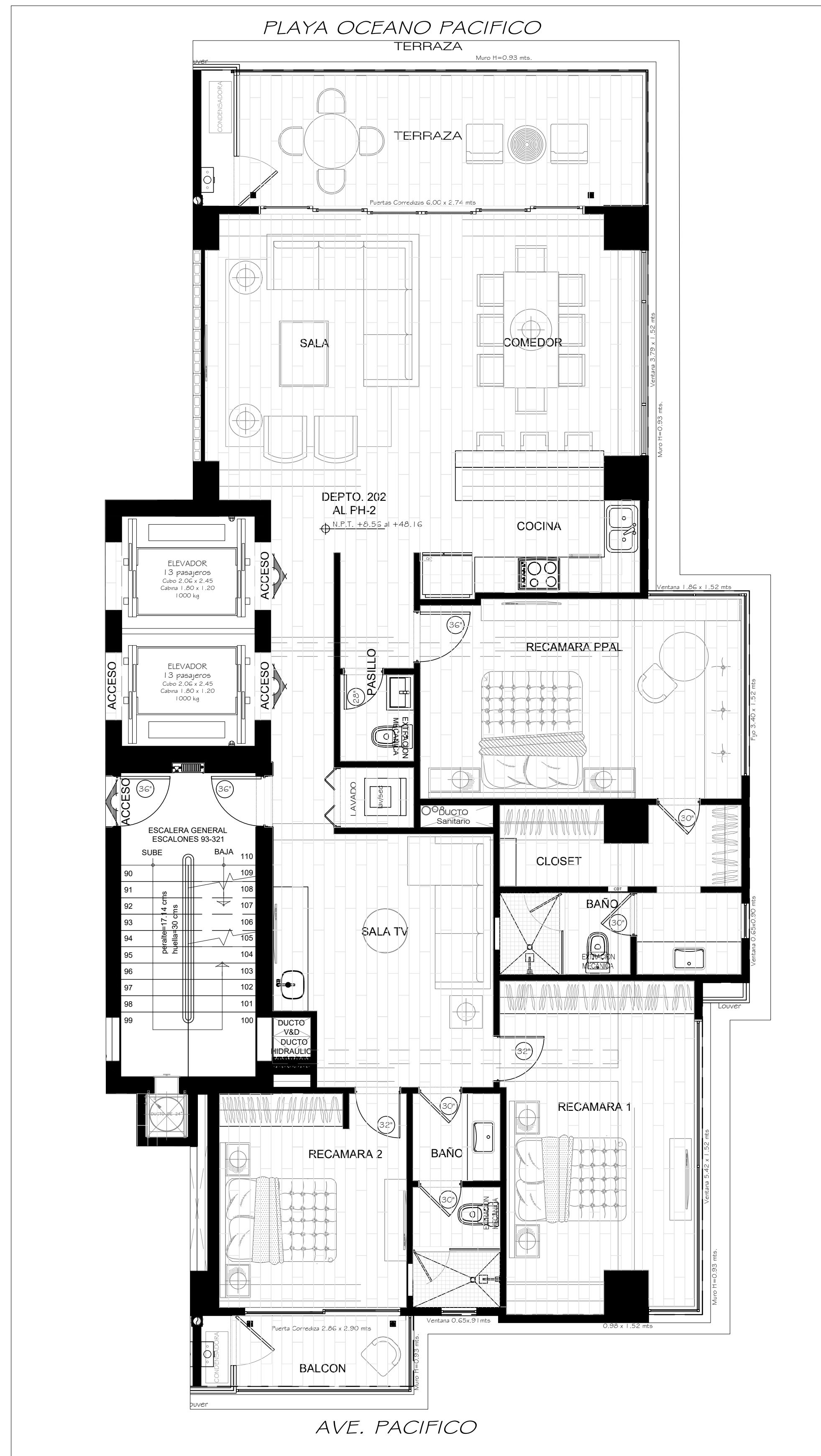
PLANTA ARQUITECTONICA DEPTO. PH2
