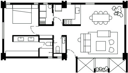
PLANTA
