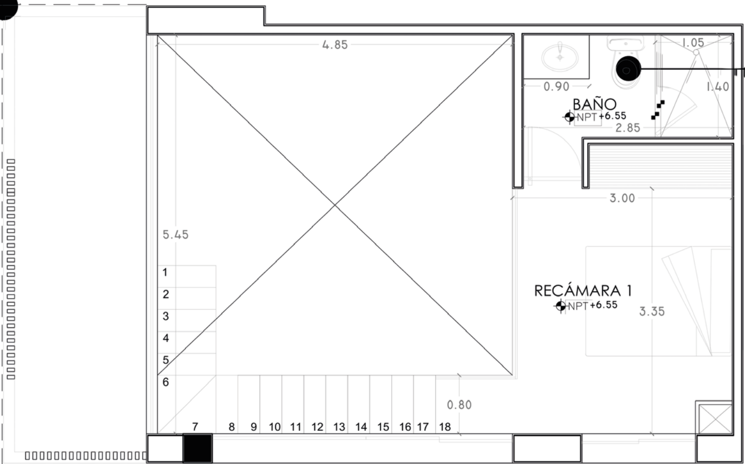
PLANTA ALTA
