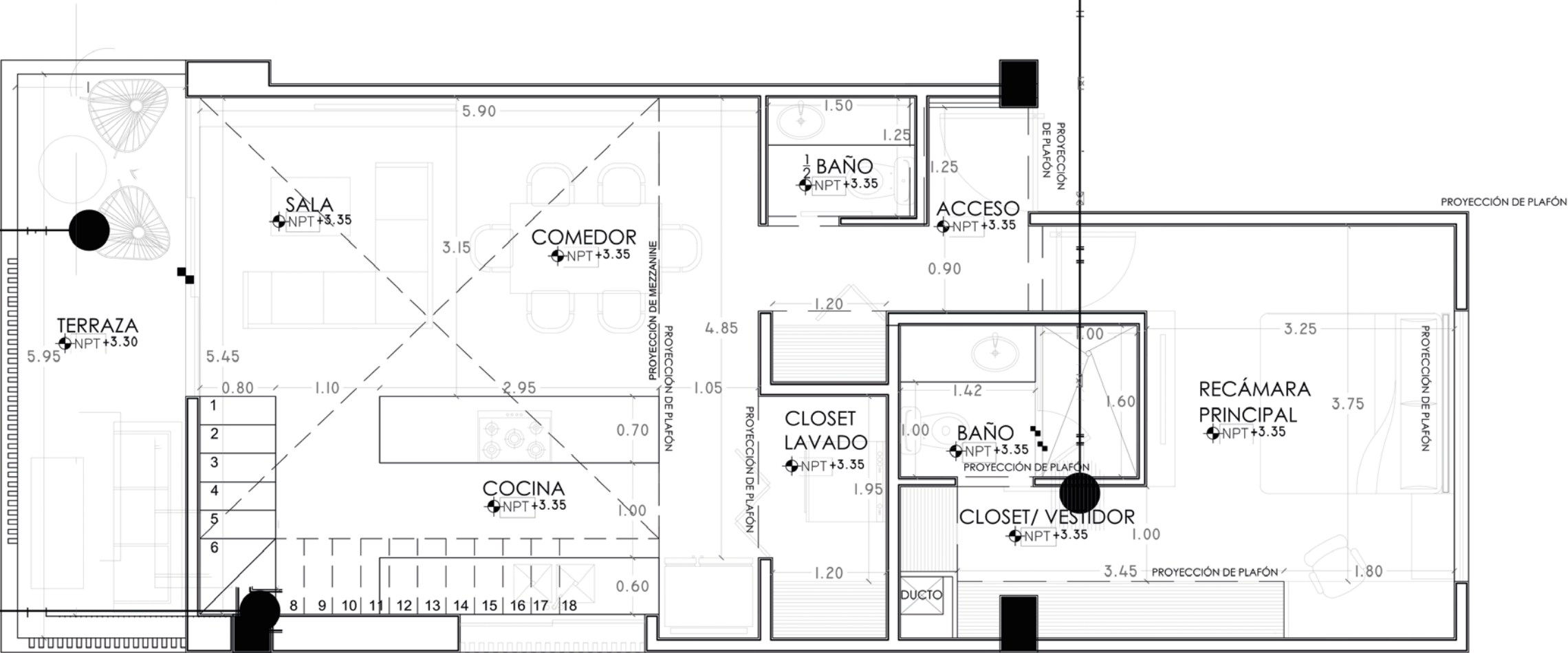
PLANTA BAJA
