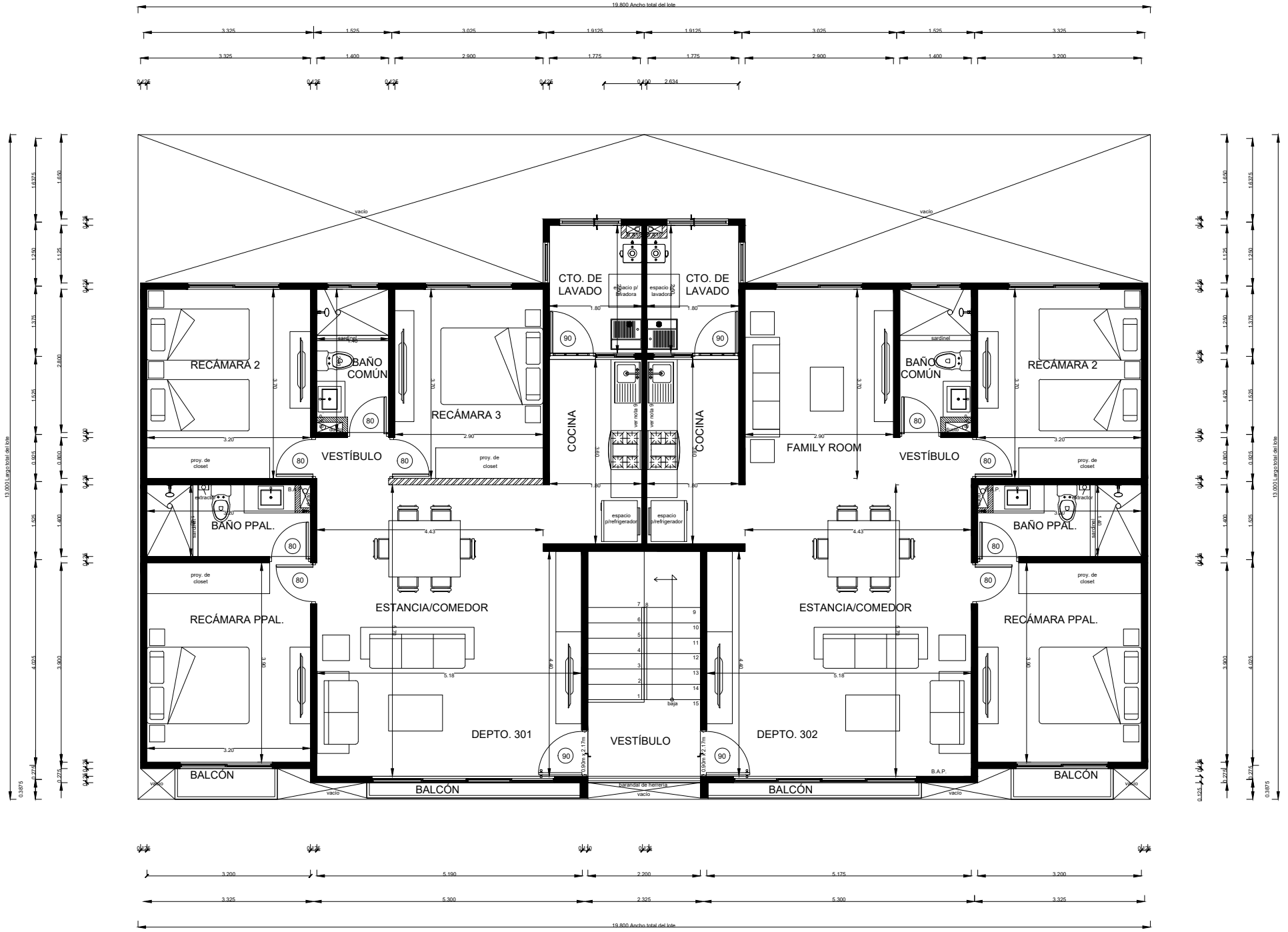
PLANTA NIVEL 3
