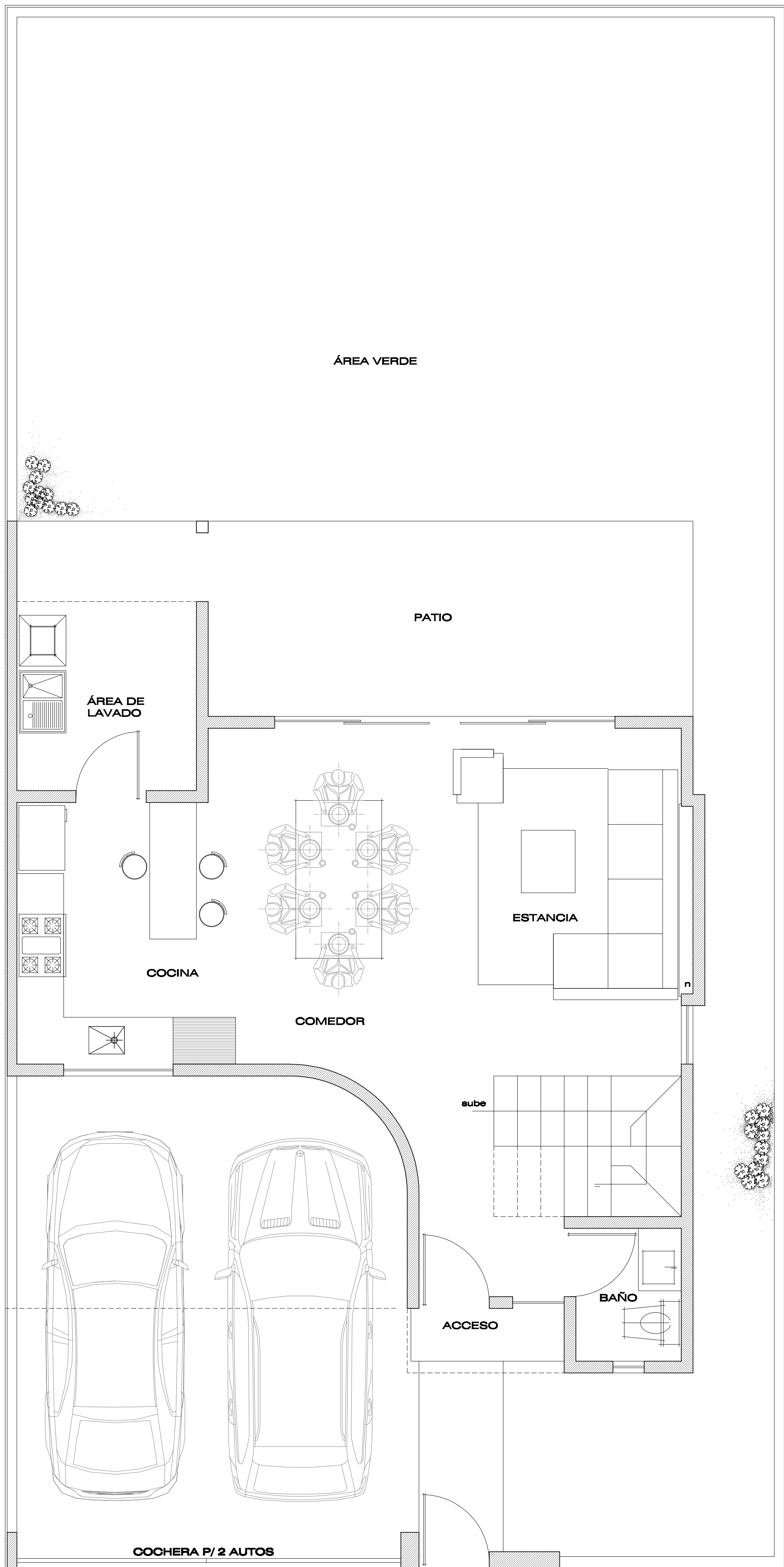
PLANTA BAJA ESCALA 1 : 7 5
