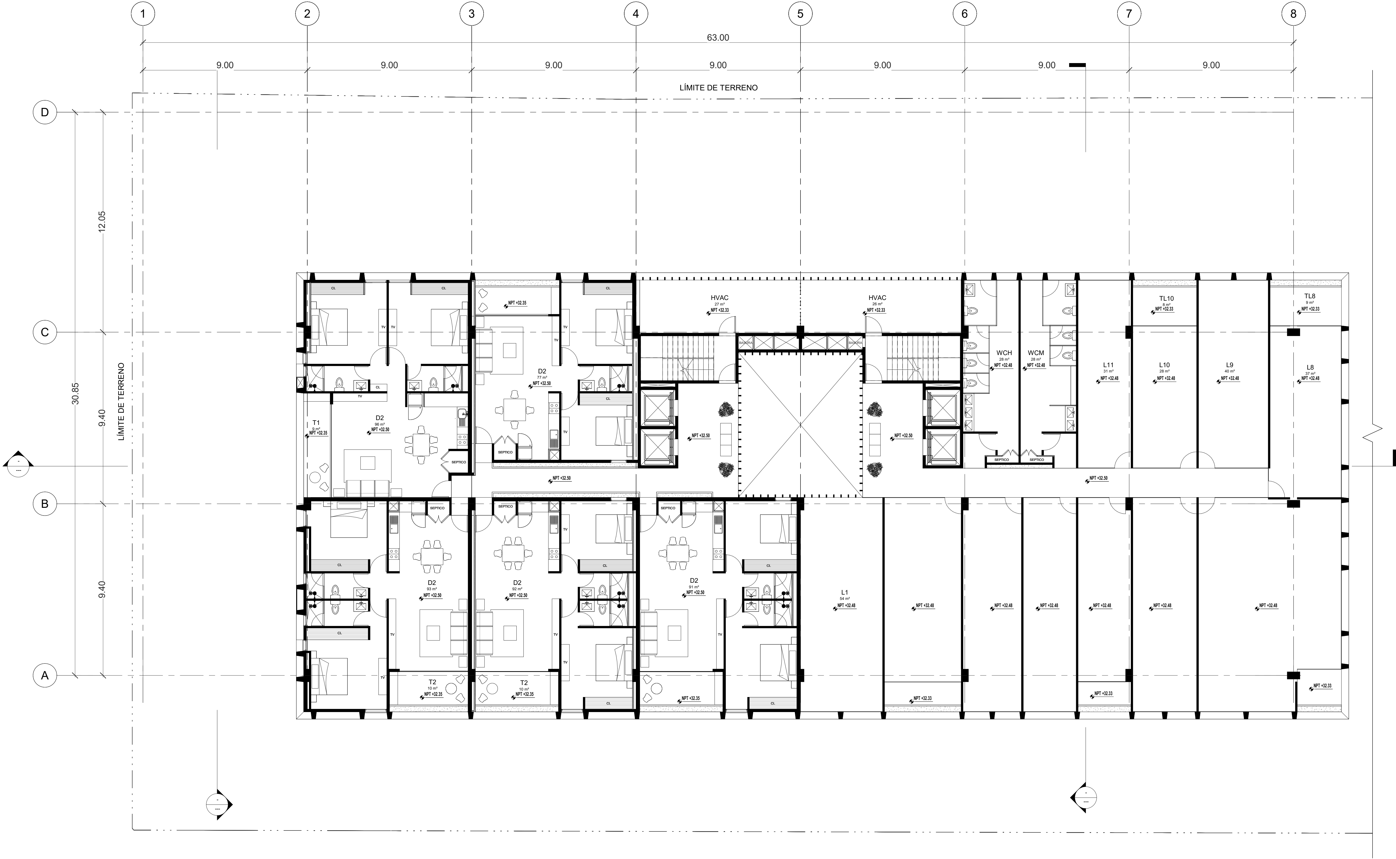
1 PLANTA NIVEL 5 1 : 100
