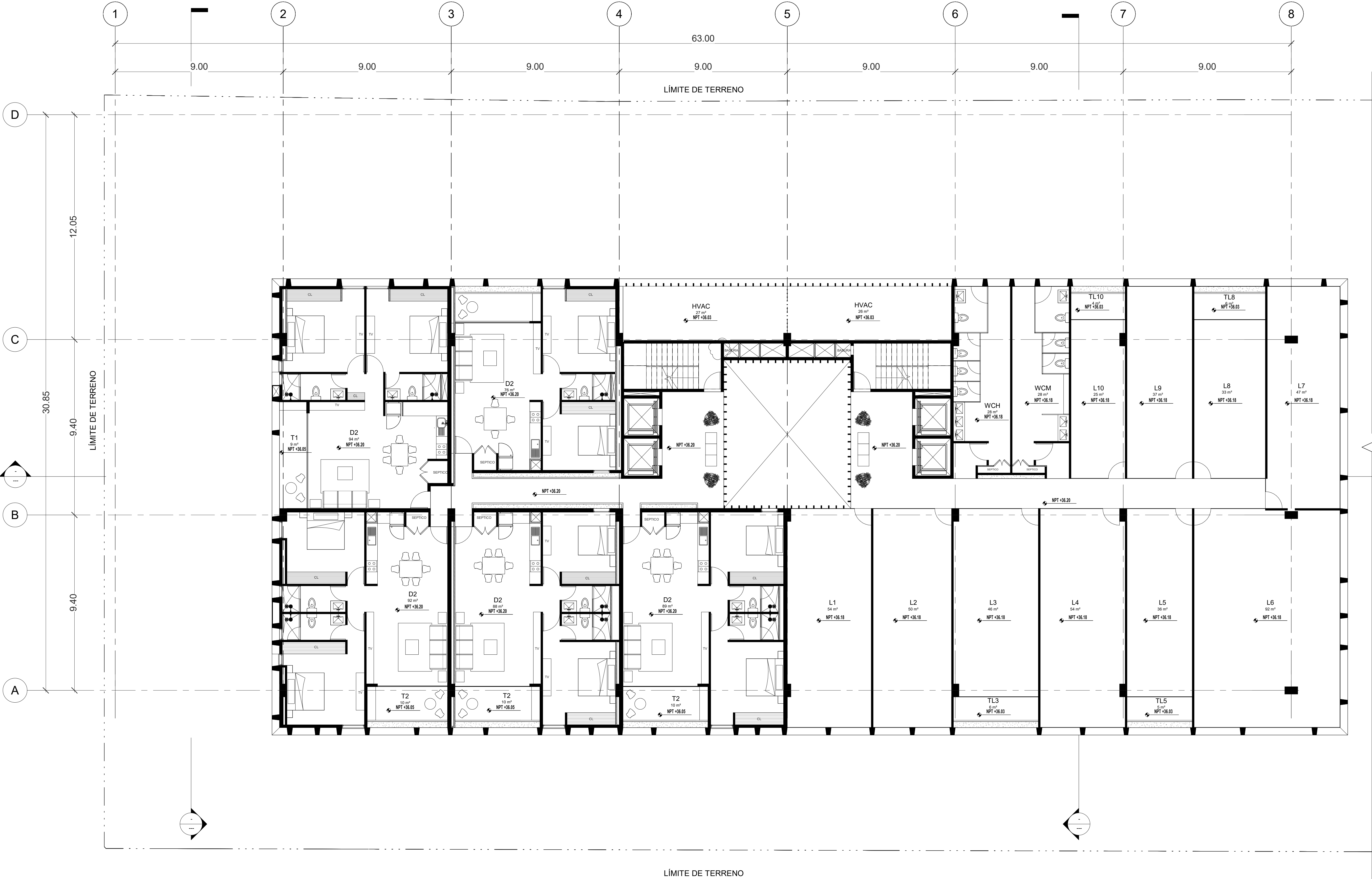
1 PLANTA NIVEL 6 1 : 100
