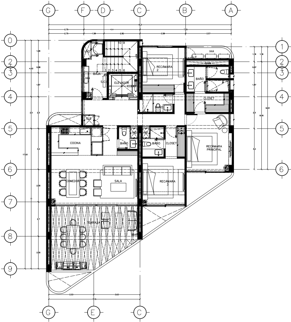
PLANTA NIVEL 11 TORRE 3
