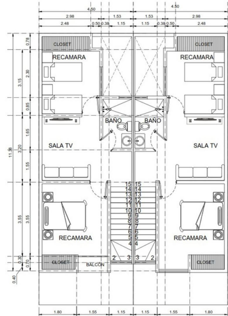
PLANTA ALTA
