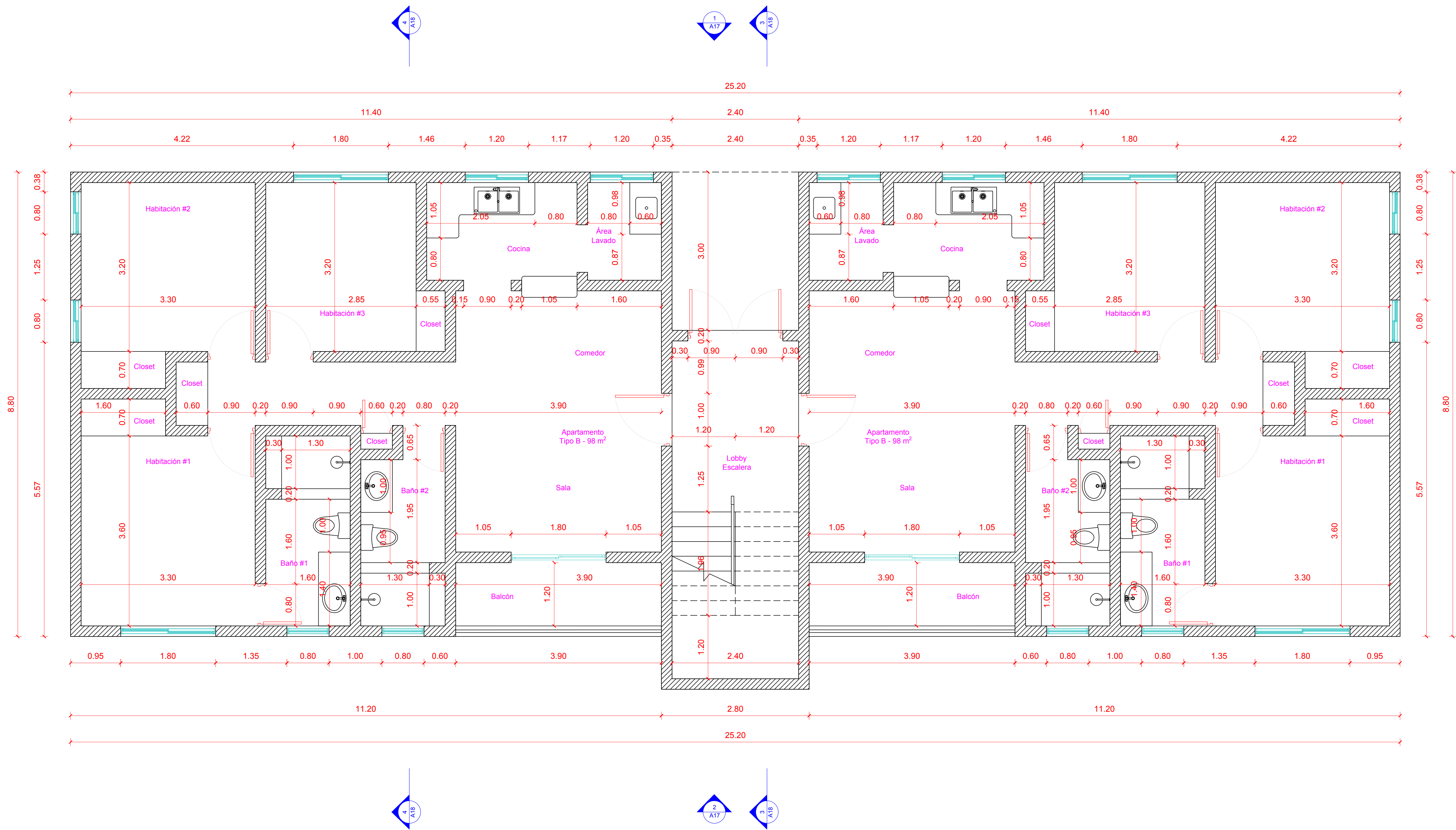
1 PLANTA DIMENSIONADA 1ER NIVEL BLOQUE TIPO B A12 Escala 1:50
