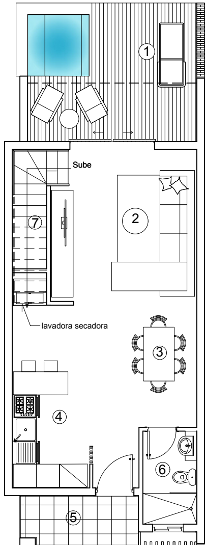
PLANTA ARQUITECTONICA 1ER. PISO
