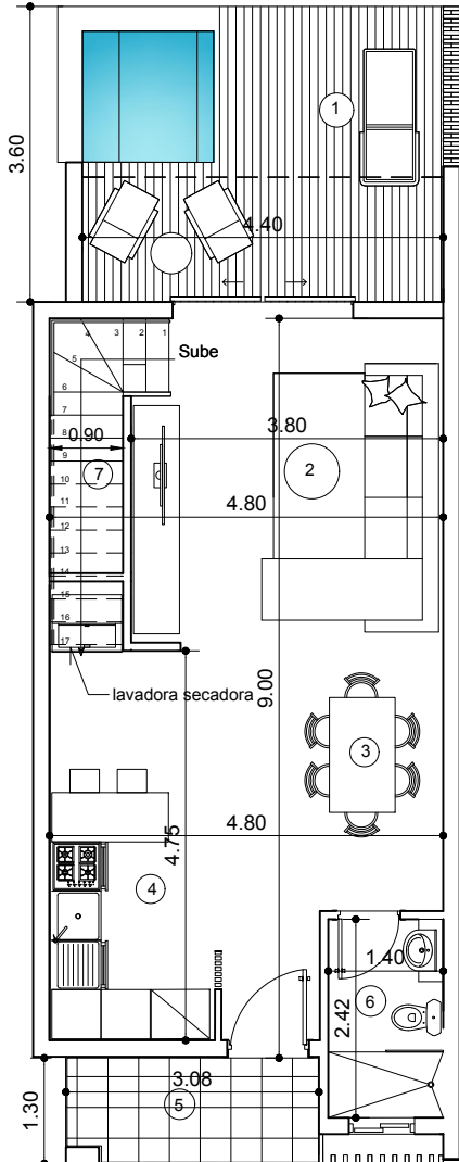
PLANTA ARQUITECTONICA 2DO. PISO
