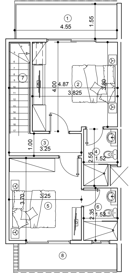
PLANTA DIMENSIONADA 2DO. PISO
