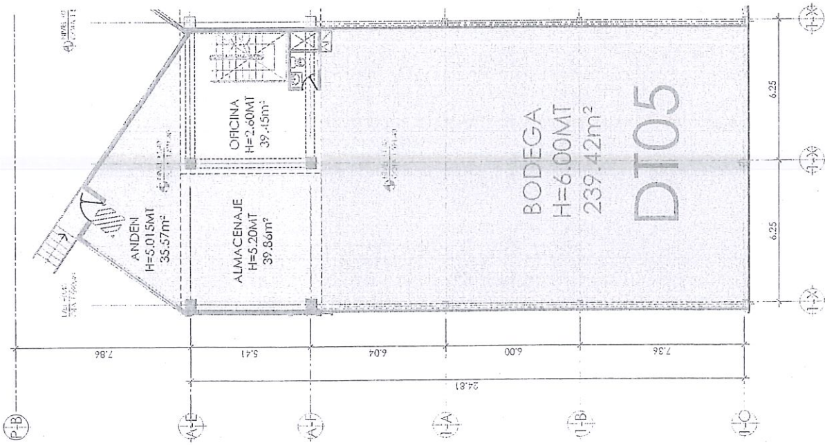
PLANTA AMUEBLADA PRIMER NIVEL DT05 SECTOR 1
