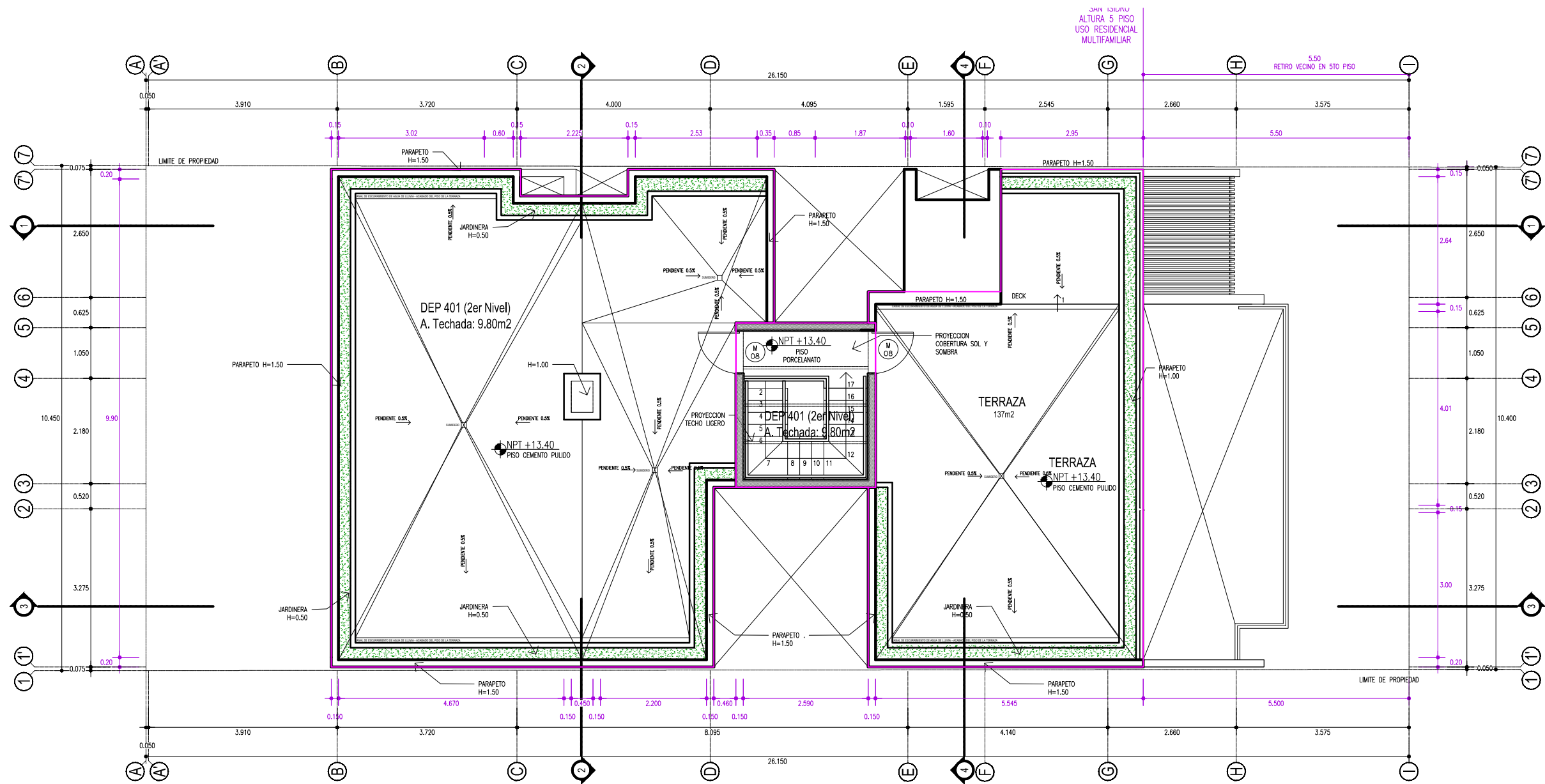
PLANTA AZOTEA ESC 1/50
