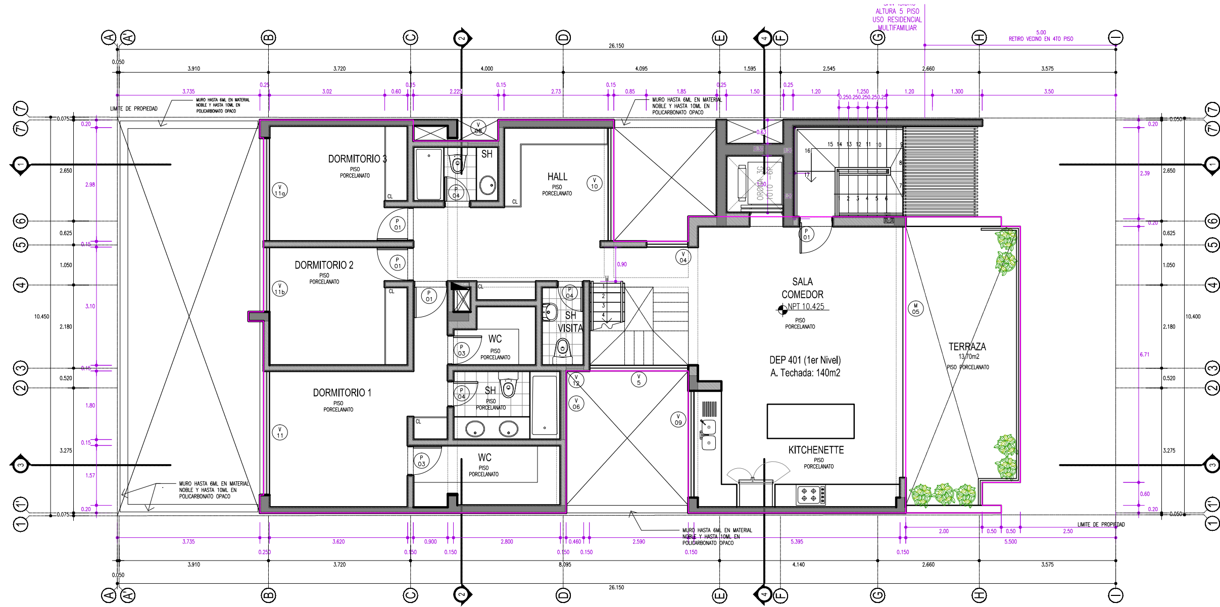
PLANTA 4TO PISO ESC 1/50
