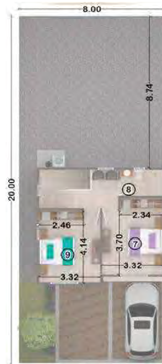
Planta Alta
