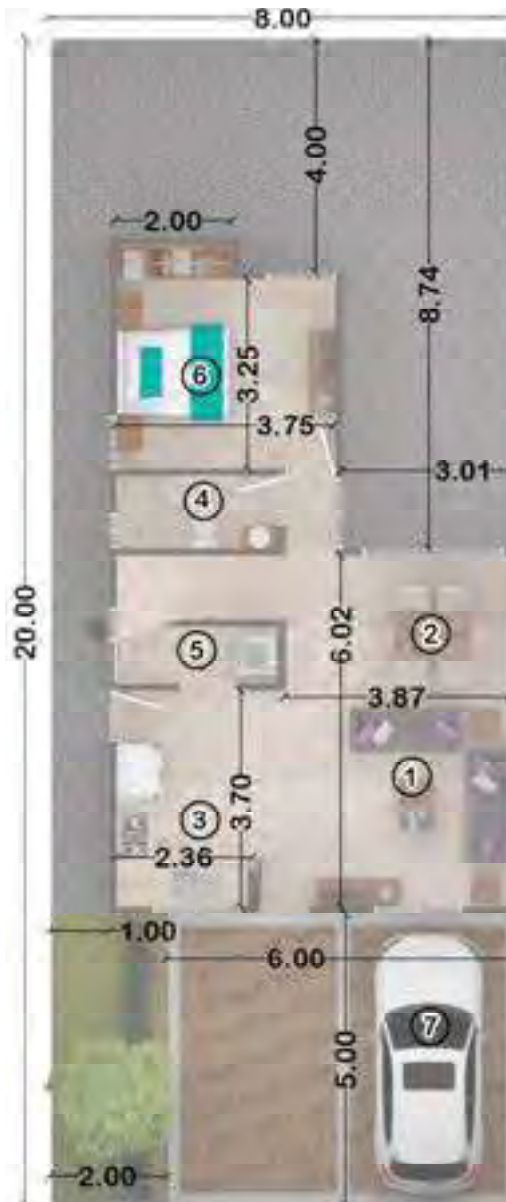
Planta Baja
