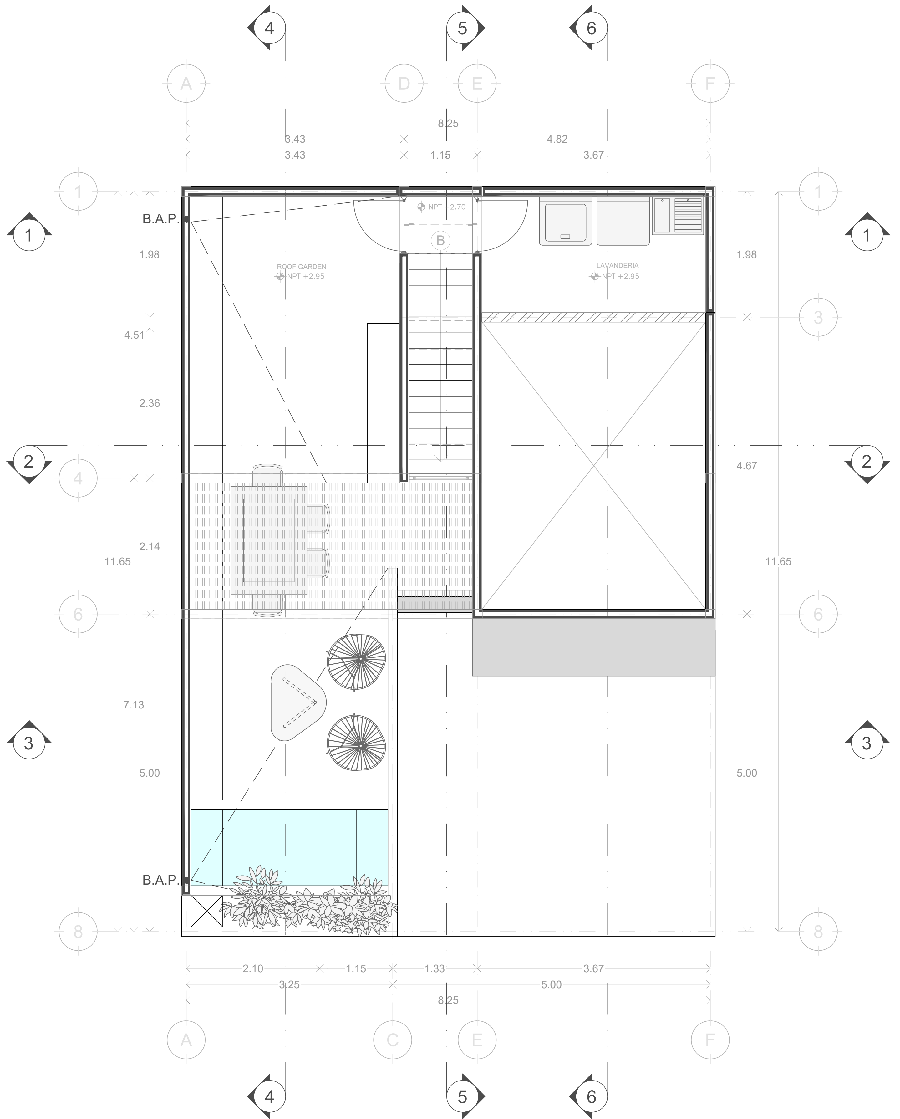
CASAS MARUVA - TIPO A PLANTA ALTA METROS
