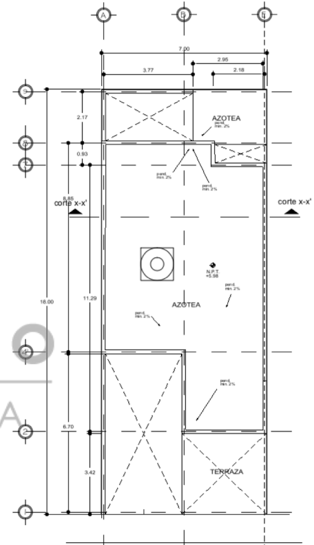
PLANTA AZOTEA
