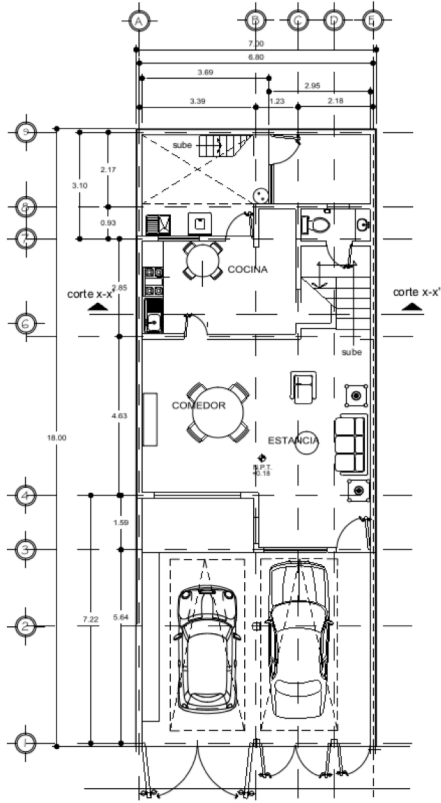
PLANTA BAJA
