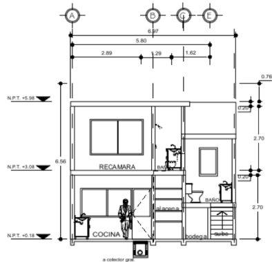
CORTE X-X'
