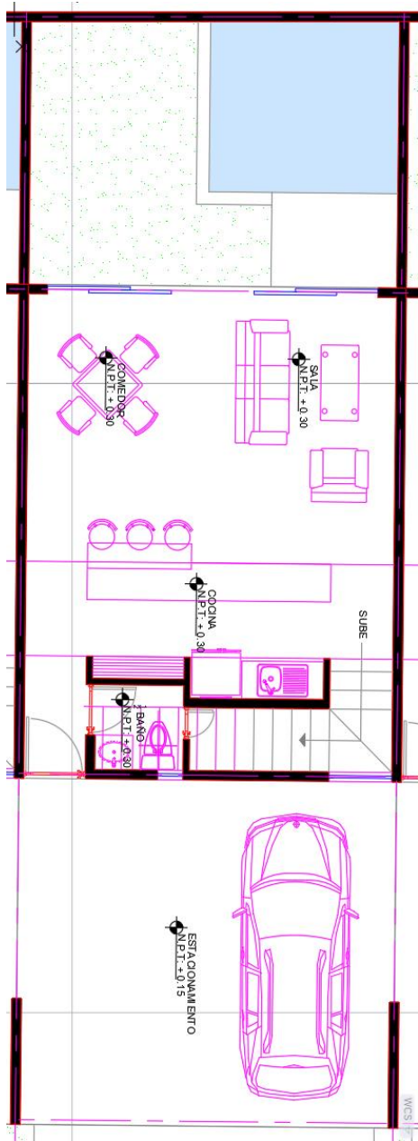
PLANTA BAJA
