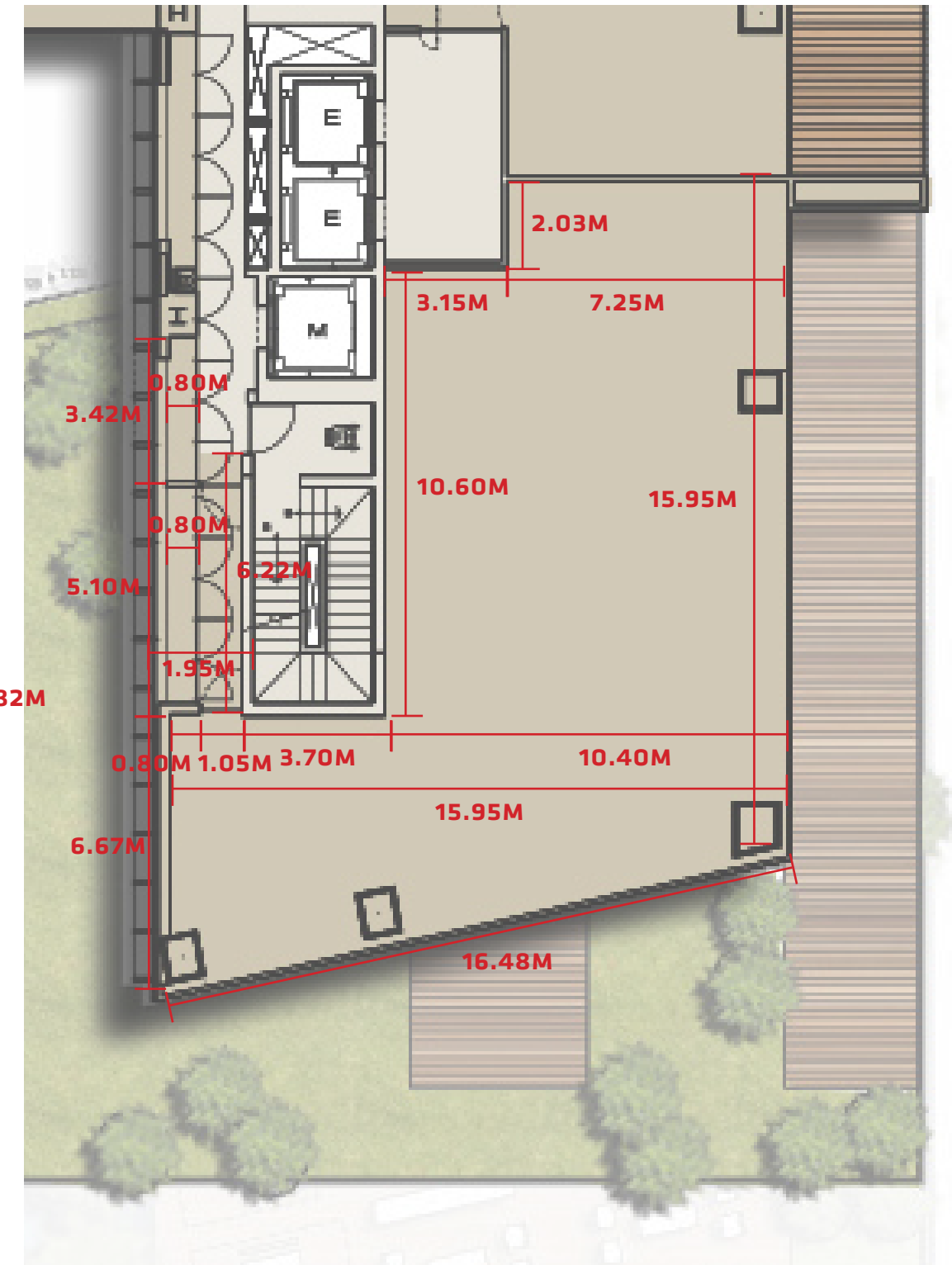
PLANTA ALTA
