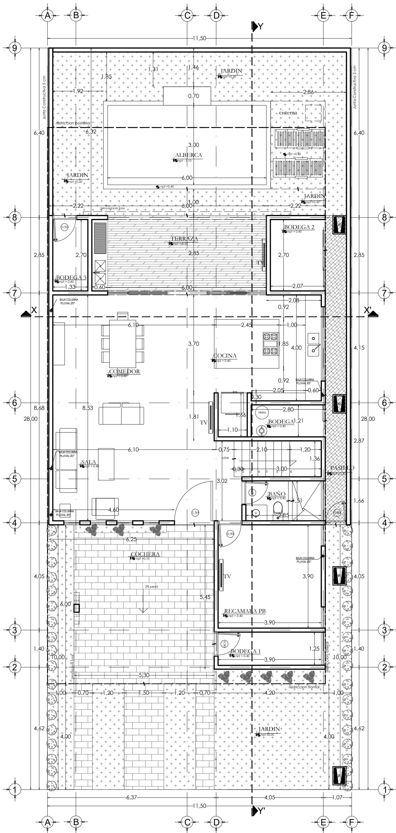
Planta baja
