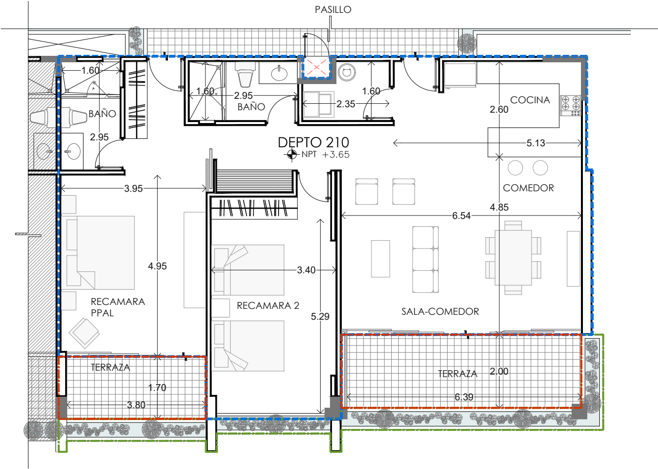
PLANTA ARQUITECTÓNICA DEPARTAMENTO 210
