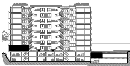
Corte del Edificio
