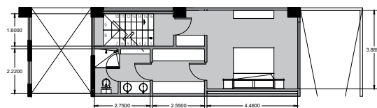
PLANTA ALTA
