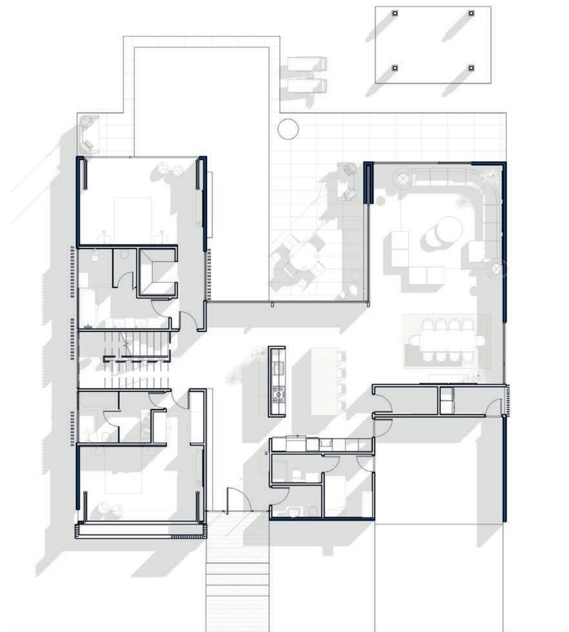
PLANTA DE ACCESO
