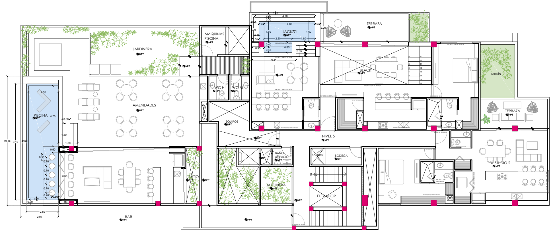
PLANTA AMENIDADES
