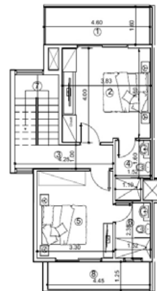
PLANTA DIMENSIONADA 2DO. PISO
