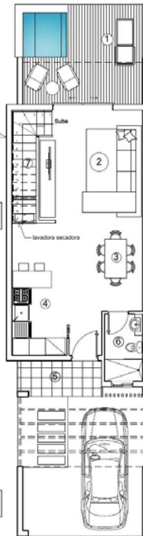
PLANTA ARQUITECTONICA 1ER. PISO
