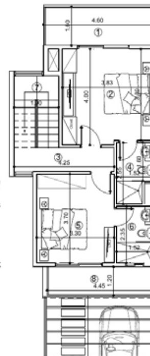
PLANTA DIMENSIONADA 2DO. PISO
