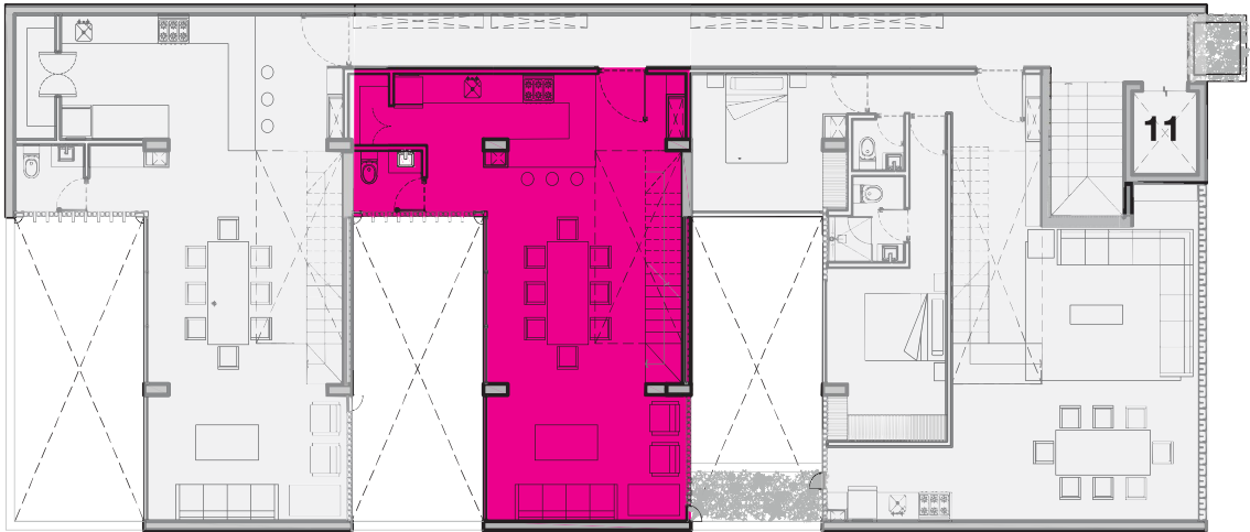
PLANTA NIVEL 04 | NIVEL +11.20
