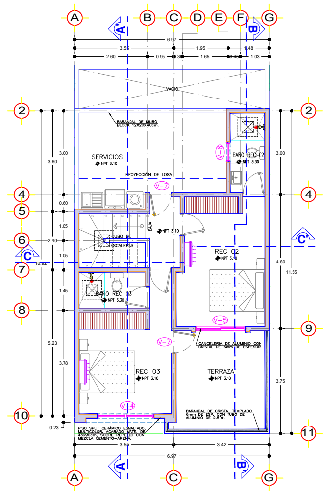
VISTA ARQUITECTÓNICA PLANTA DE ENTREPISO
