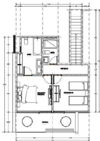
PLANTA 2da. NIVEL SANTOS TULUM
