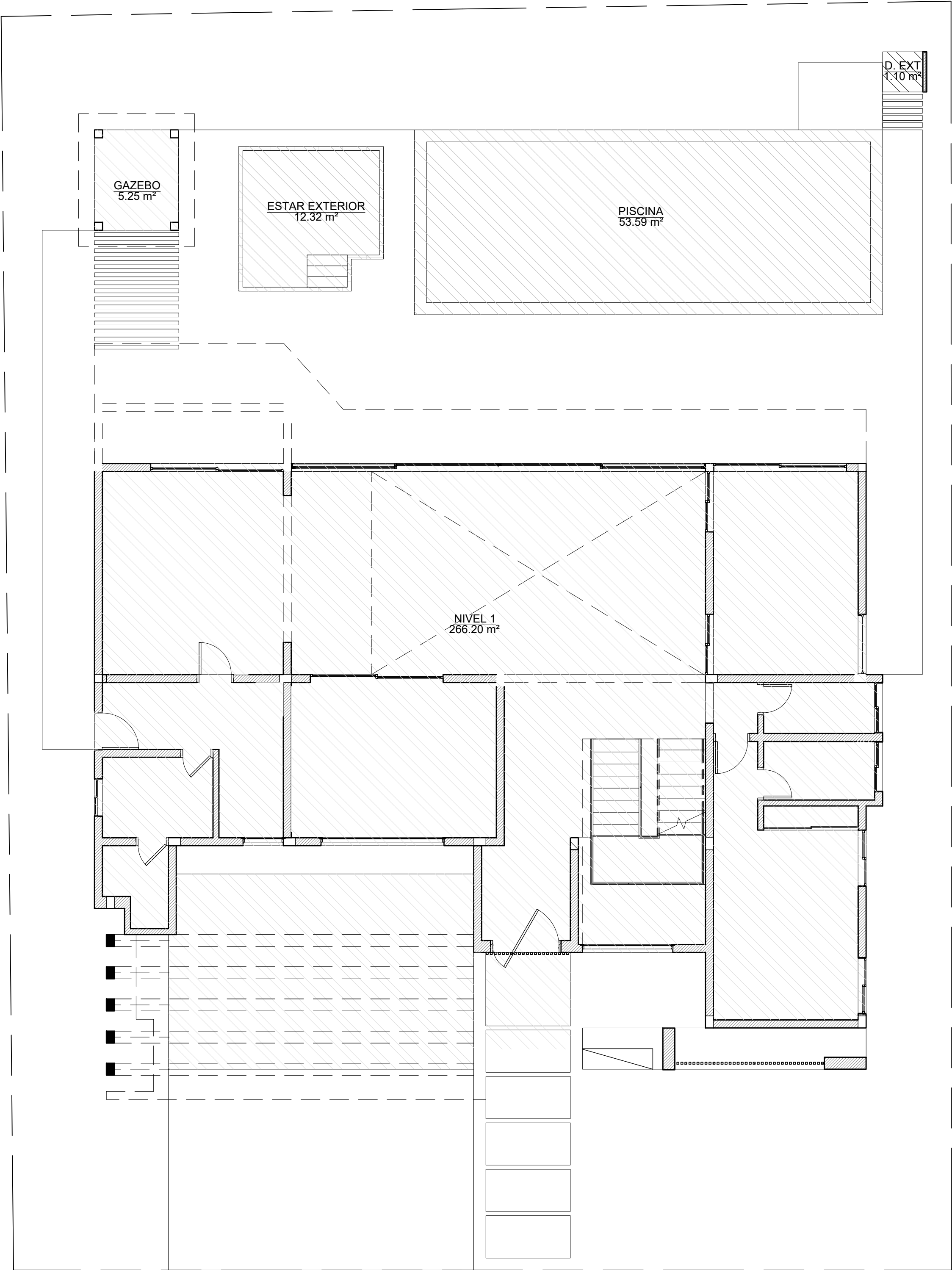
1 PLANO M2 NIVEL 1 ESC. 1 : 100
