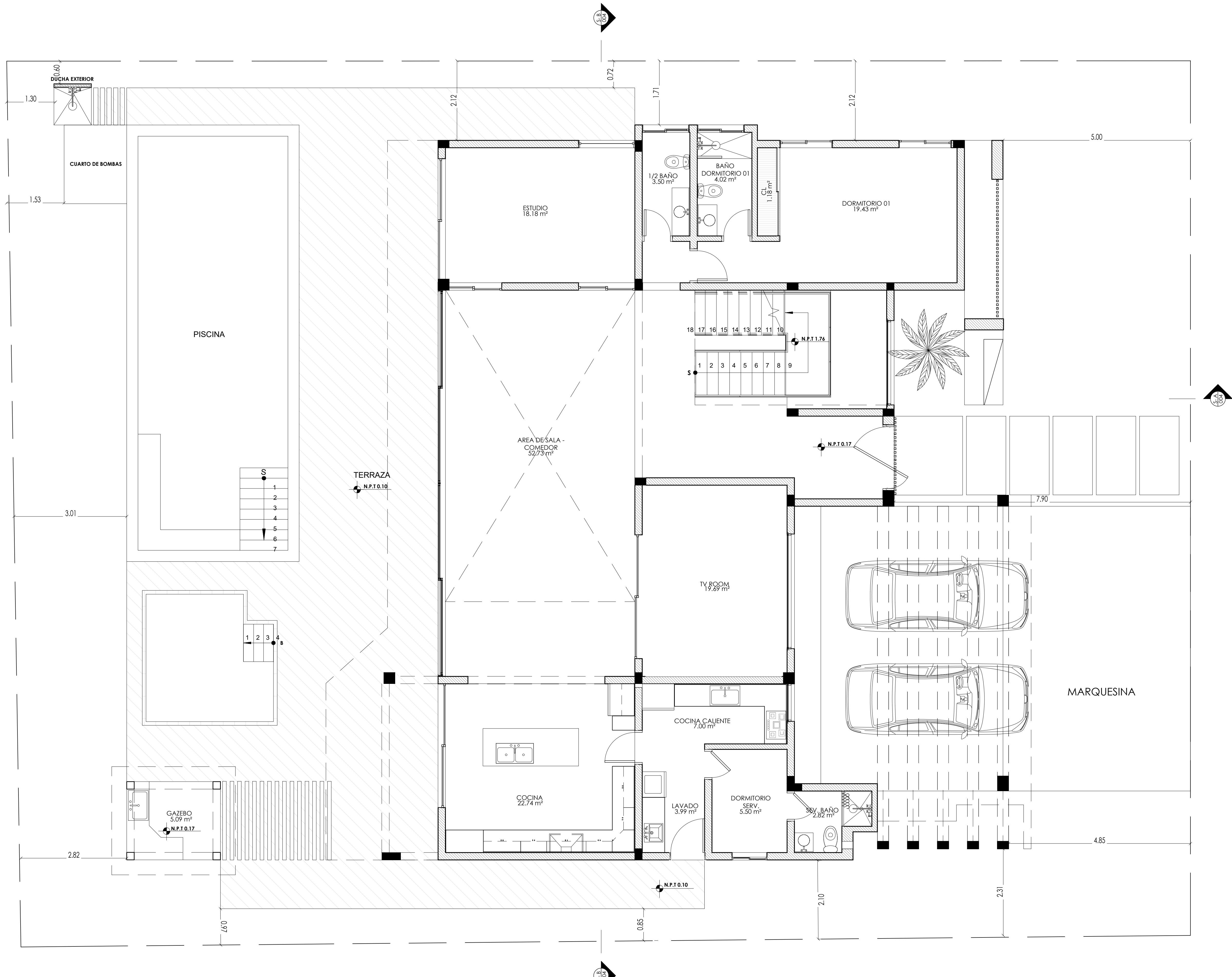
1 PLANTA DE LINDEROS ESC 1 : 50
