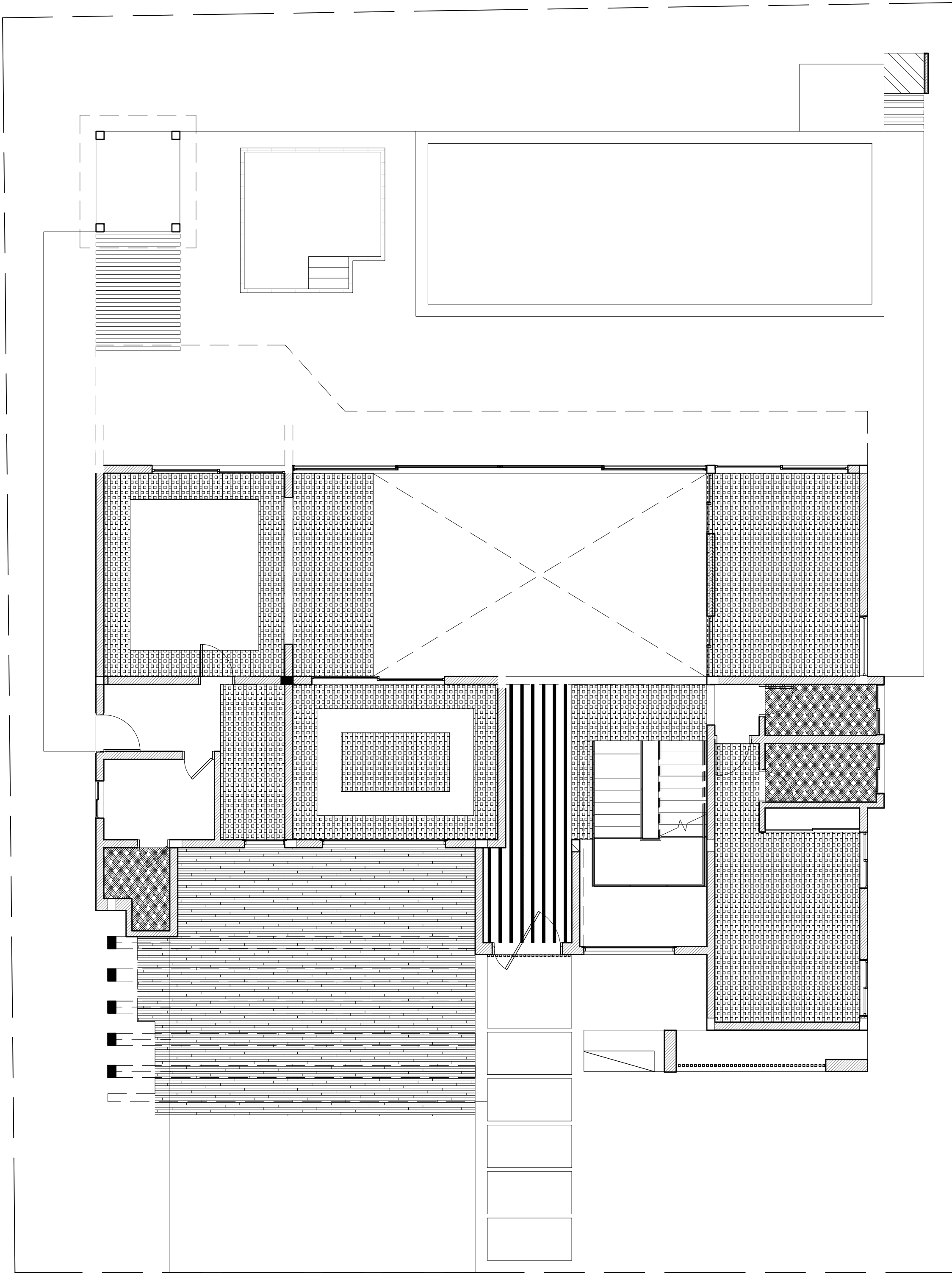
1 PLANO DE PLAFONES NIVEL 1 ESC 1:100
