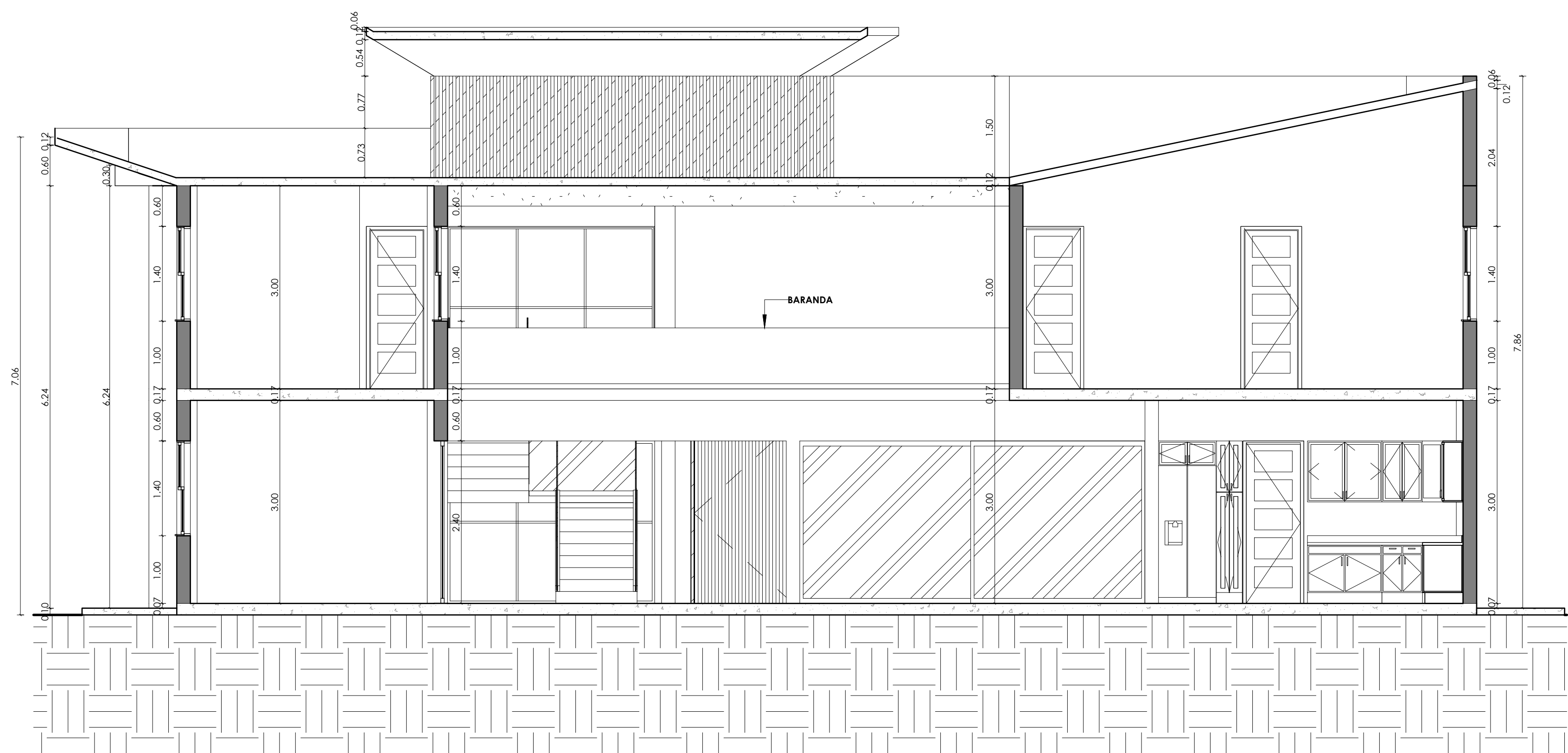
2 SECCION-B ESC 1:50
