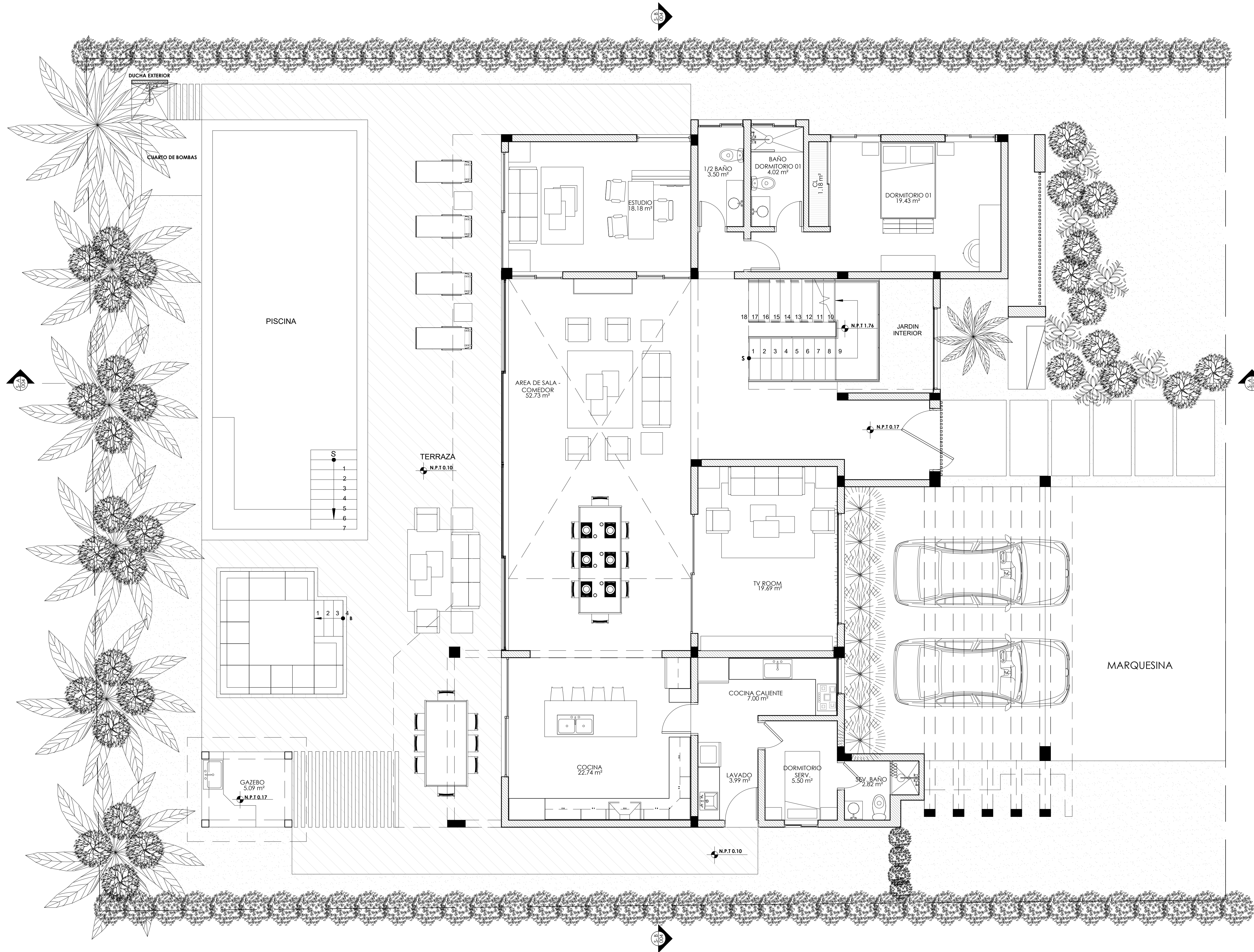
1 PLANO DE CONJUNTO ESC. 1 : 50
