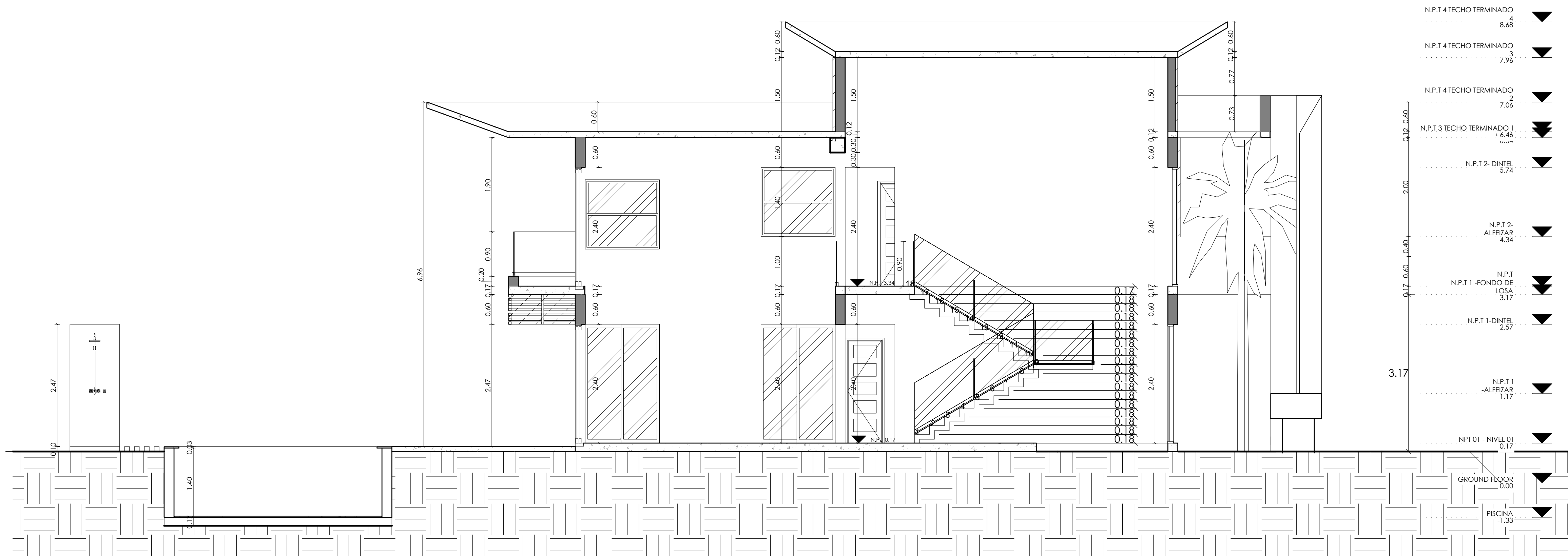
1 SECCION-A ESC 1:50
