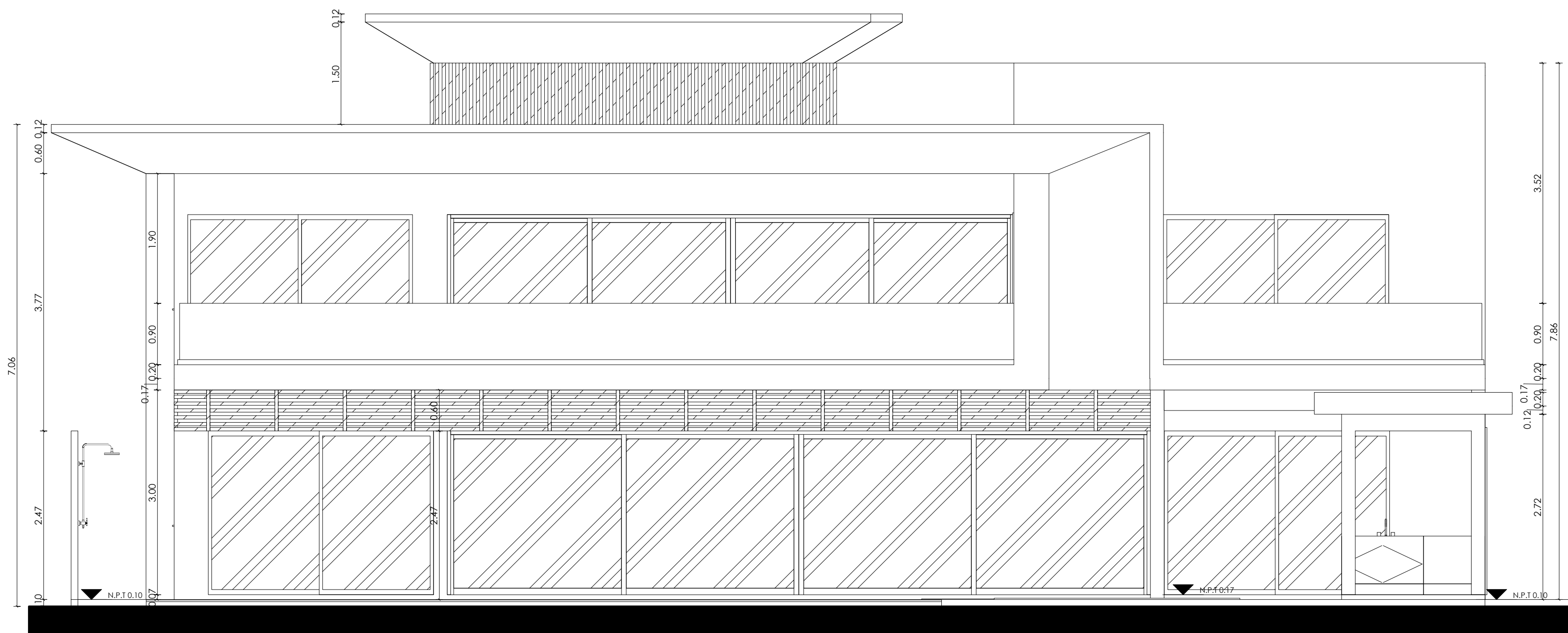
8 ELEVACION POSTERIOR ESC 1 : 50
