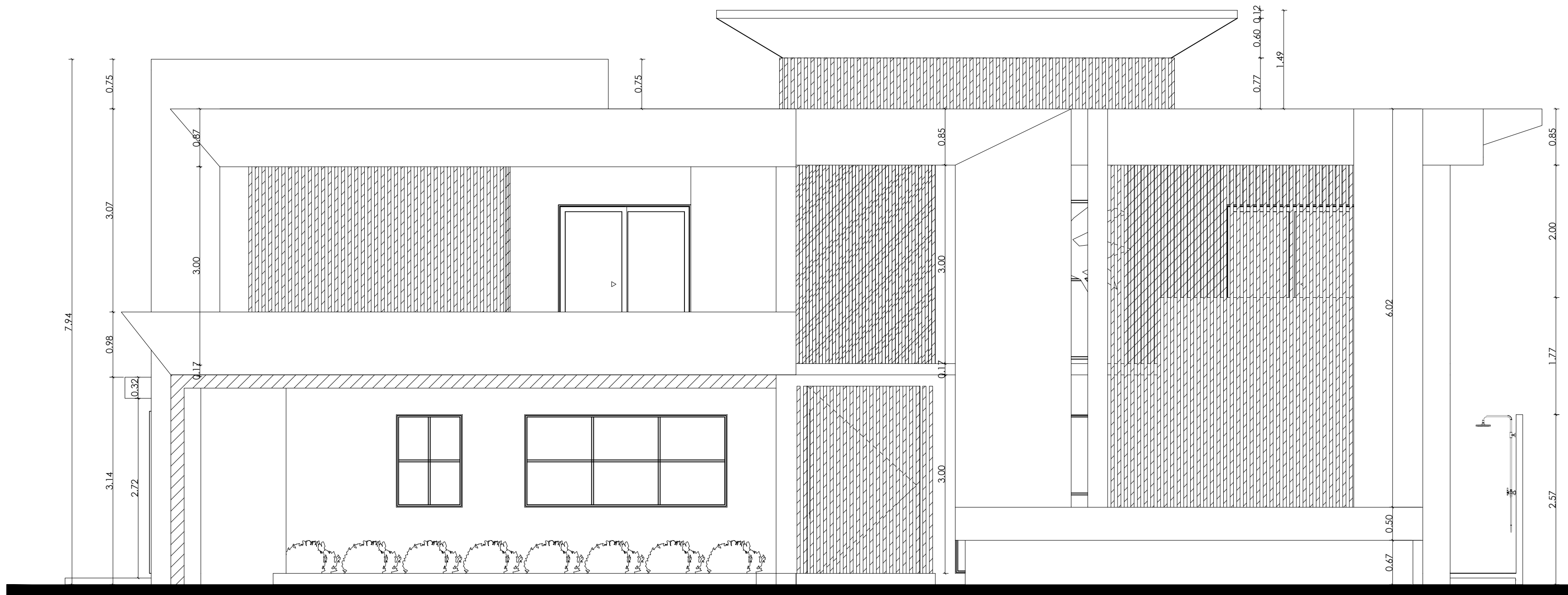
1 ELEVACION FRONTAL ESC 1 : 50
