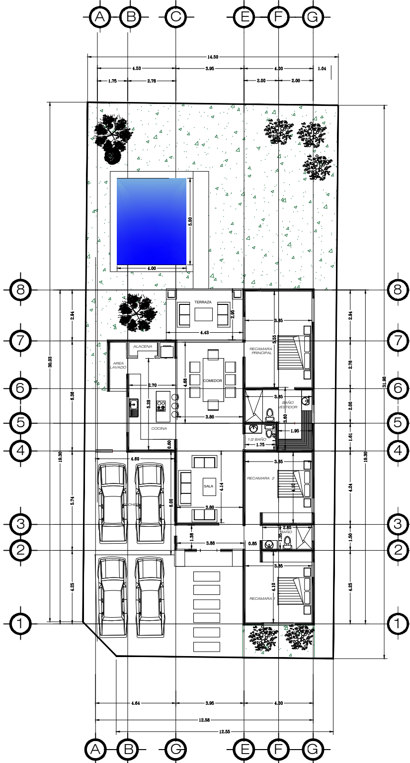
PLANTA BAJA
