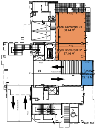
PLANTA BAJA
