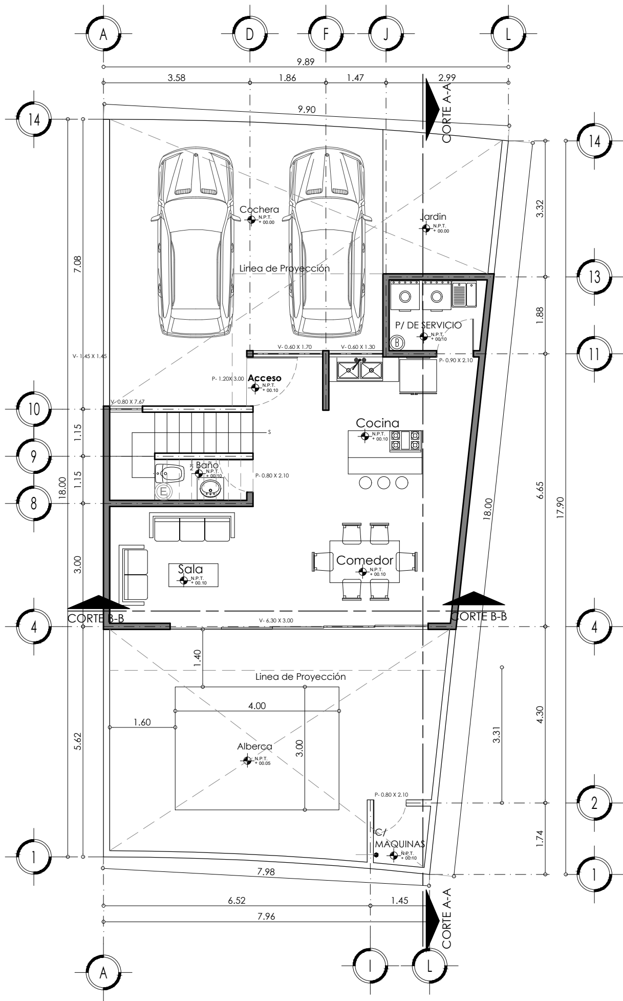
PLANTA ARQUITECTONICA BAJA 61.19 M2 DE CONSTRUCCIÓN
