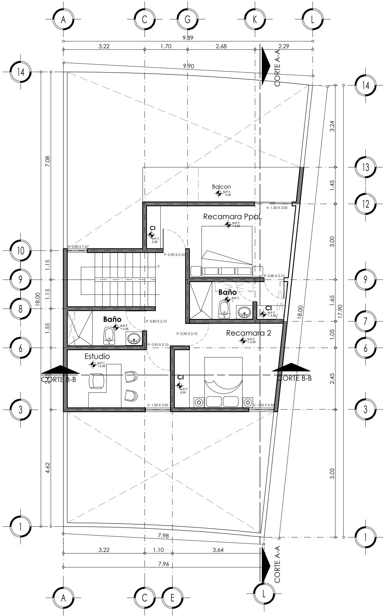
PLANTA ARQUITECTONICA ALTA 60.03 M2 DE CONSTRUCCIÓN
