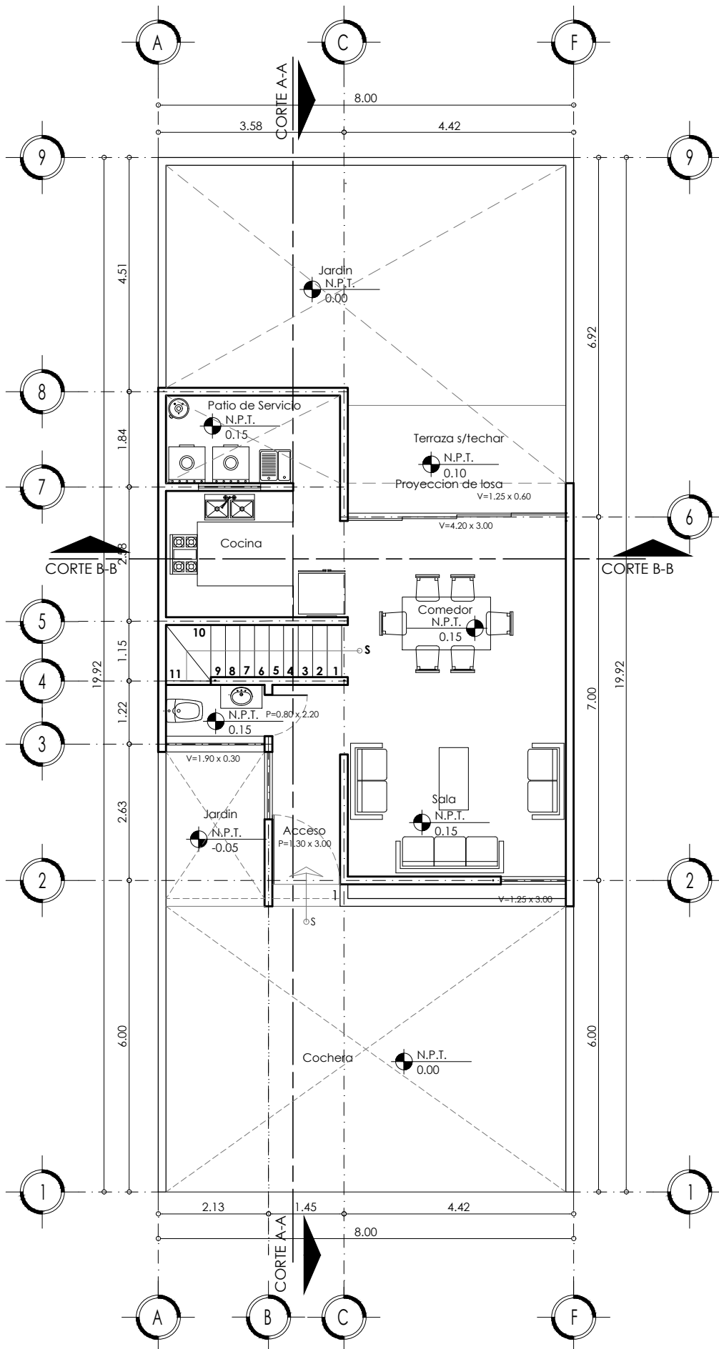
PLANTA ARQUITECTONICA BAJA SUP. DE CONSTRUCCION 54.30M2
