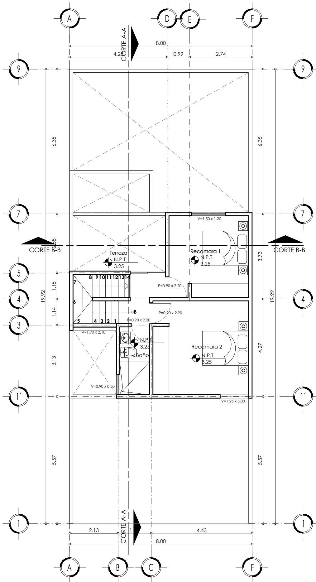
PLANTA ARQUITECTONICA ALTA SUP. DE CONSTRUCCION 42.01 M2
