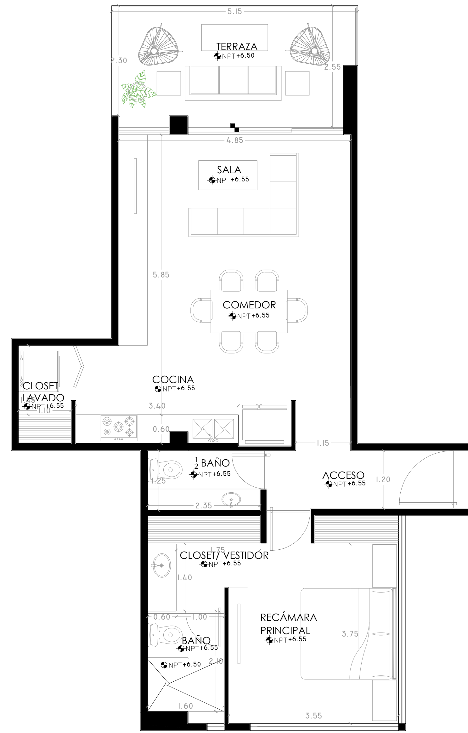
PLANTA BAJA
