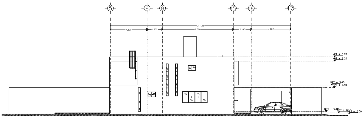
FACHADA LATERAL IZQUIERDO
