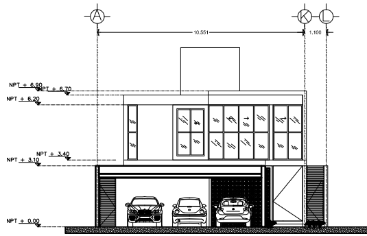
FACHADA FRONTAL
