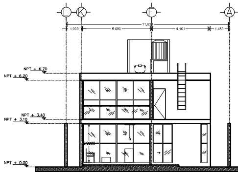
FACHADA POSTERIOR
