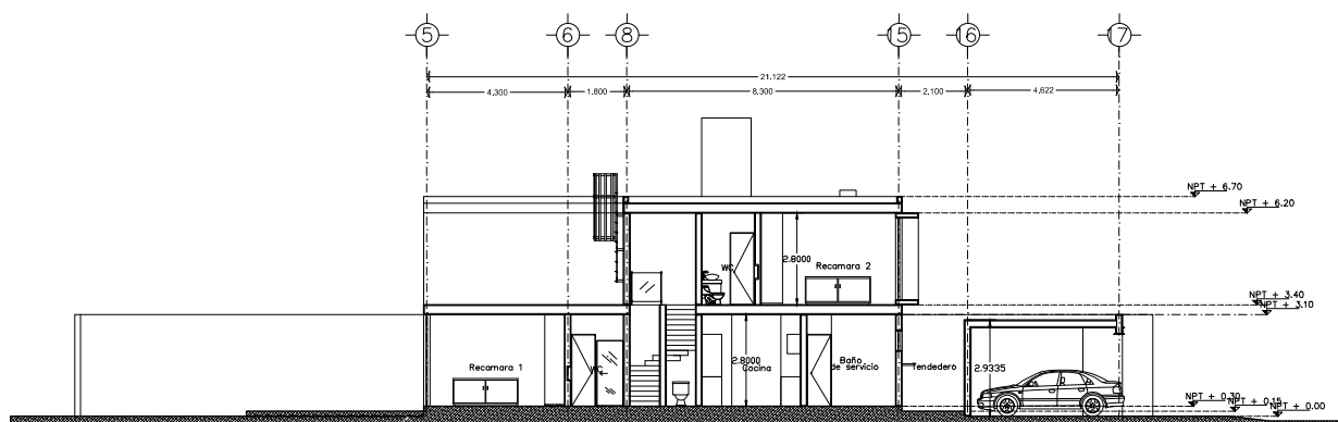
CORTE 4 - 4'
