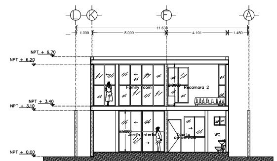
CORTE 3 - 3'
