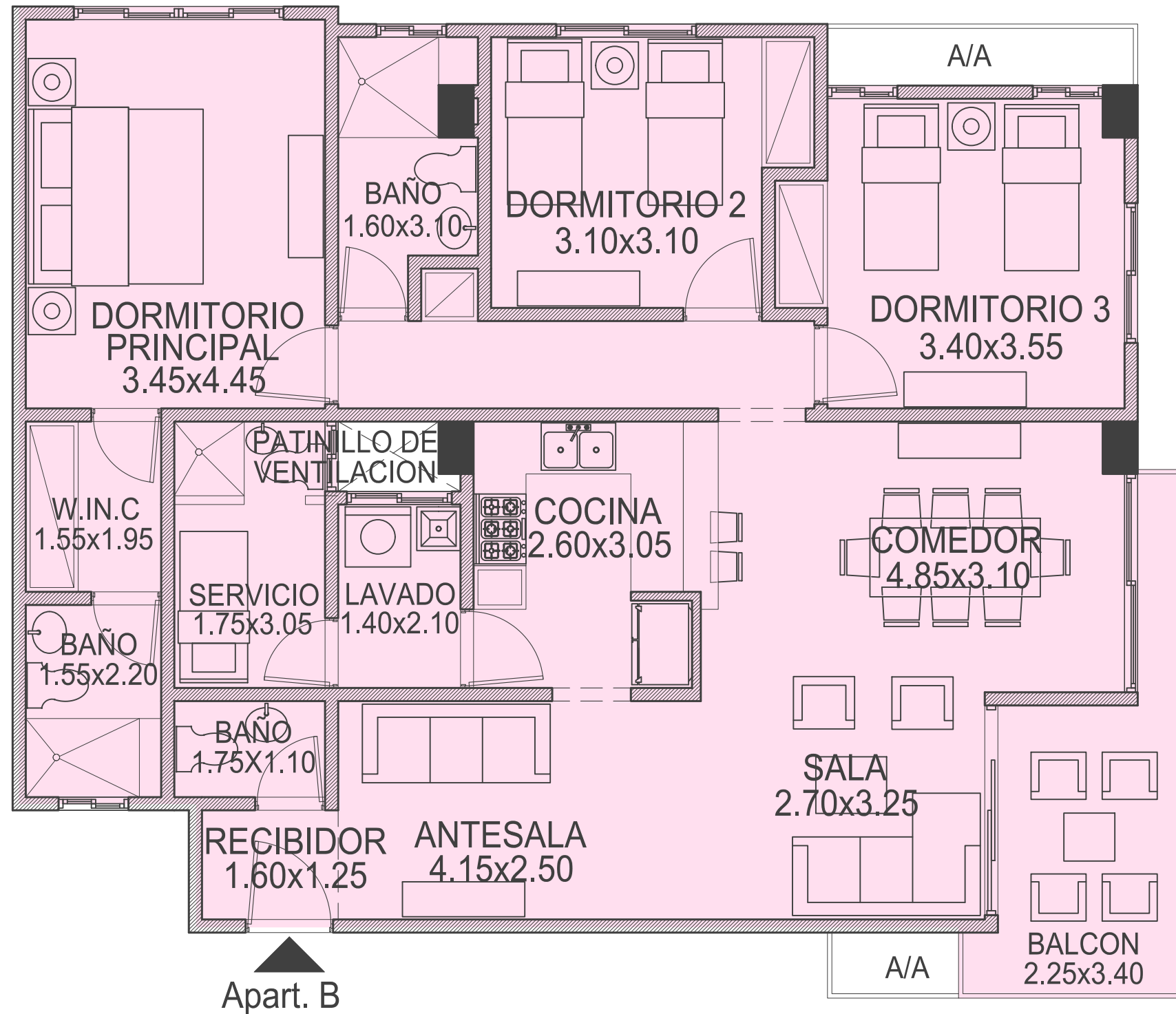
APARTAMENTO B Y E 133.2760 m 2
