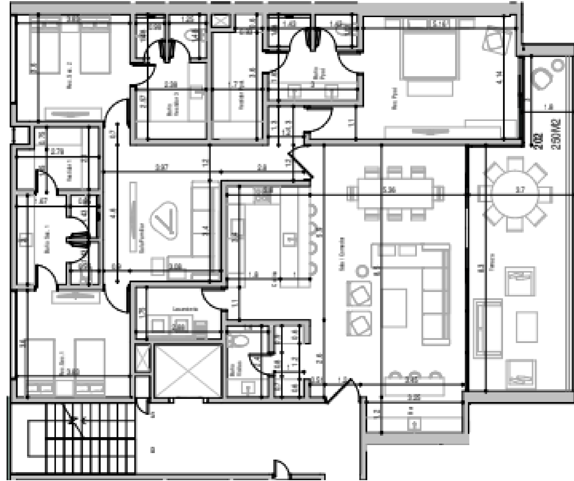
1 DEPARTAMENTO 202 1 : 100
