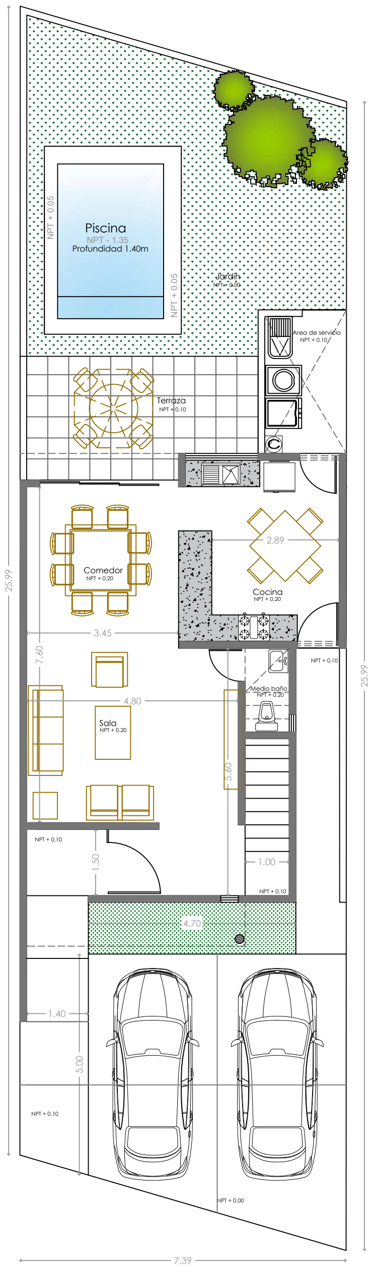
PLANTA BAJA
